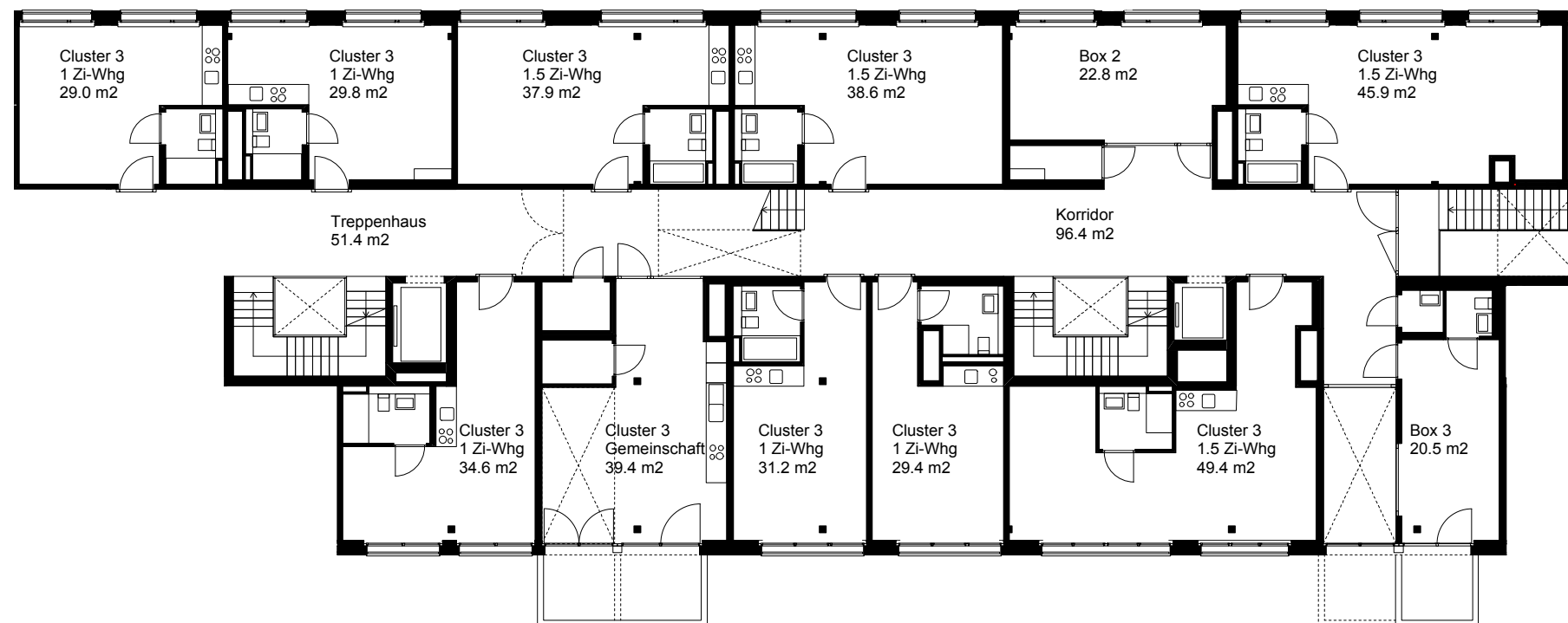
GRUNDRISS WOHNCLUSTER 3 1:200
