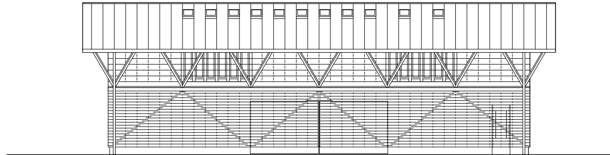
Westfassade Holzatelier, Ersatzneubauten Lüssihof
