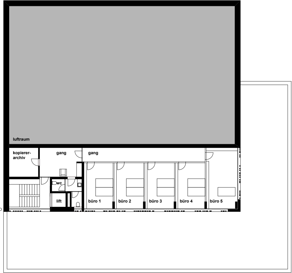
3. obergeschoss
