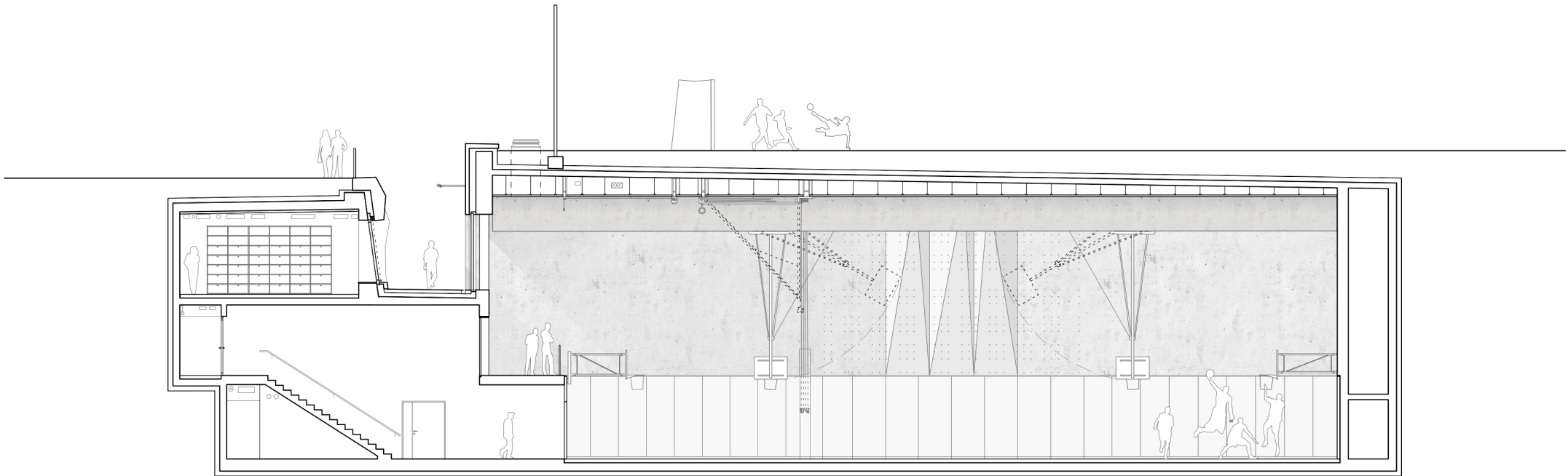
Schnitt 4-4
