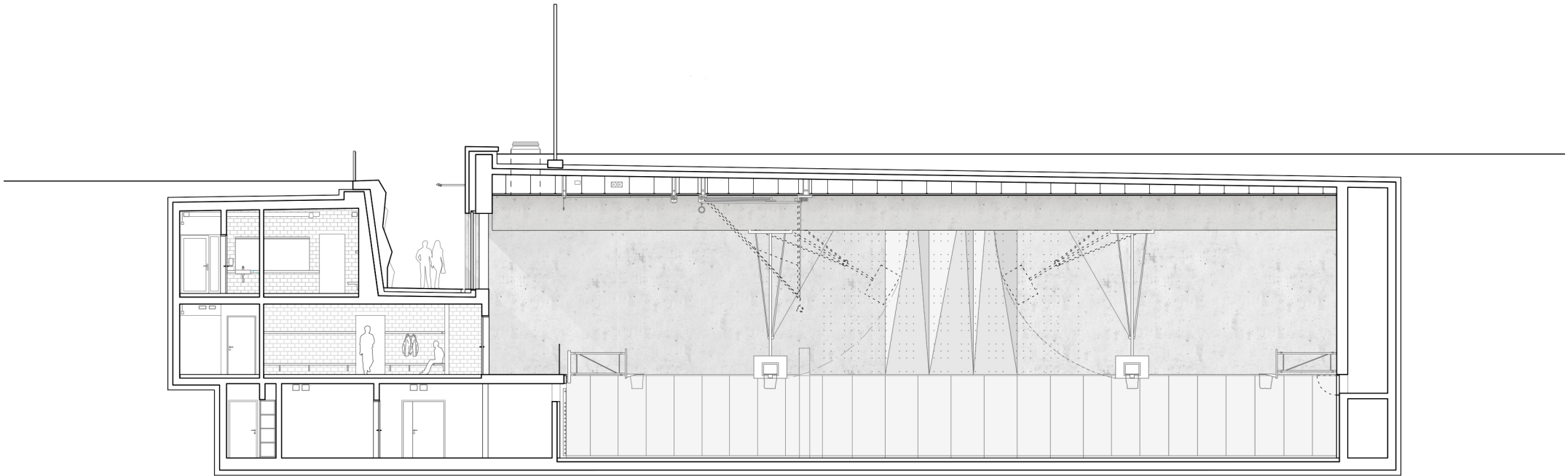
Schnitt 3-3
