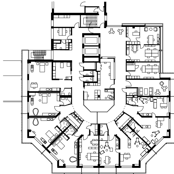
3. OG Frauenklinik Gebärzimmer / Ambulatorium
