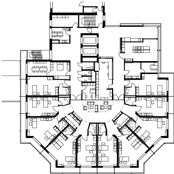
2. OG Frauenklinik Pflegeabteilung
