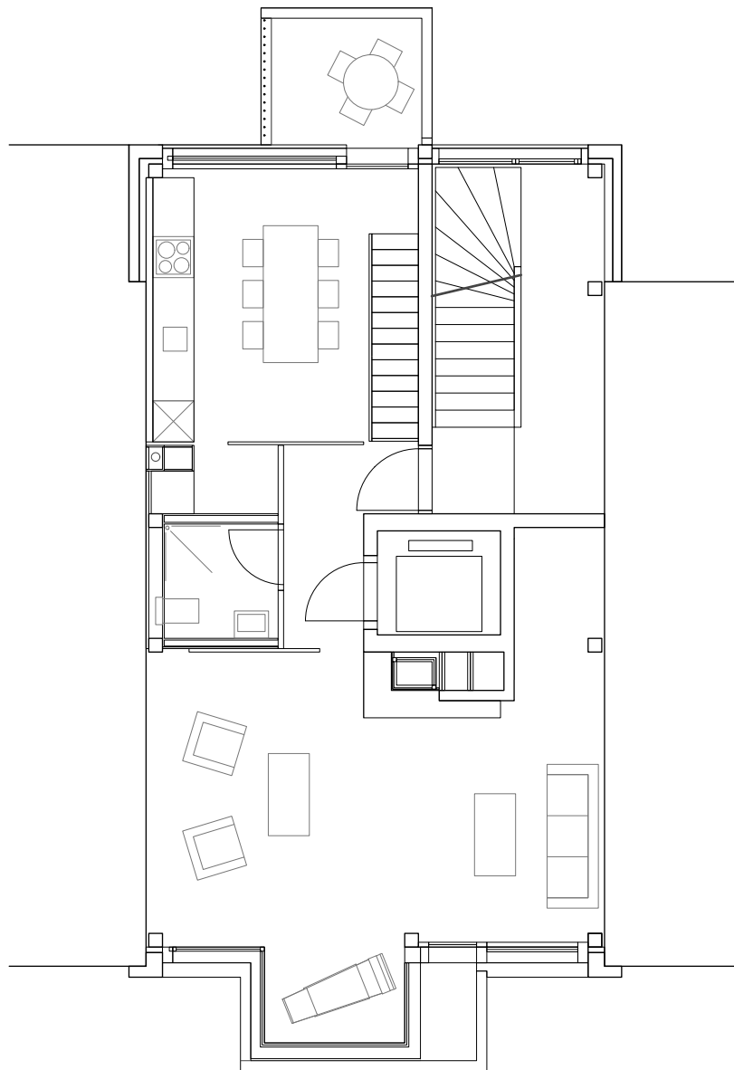
2. Obergeschoss 1:100
