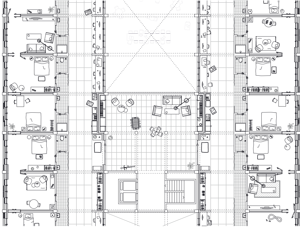
Plan 10: Eingangsbereich 1:50
