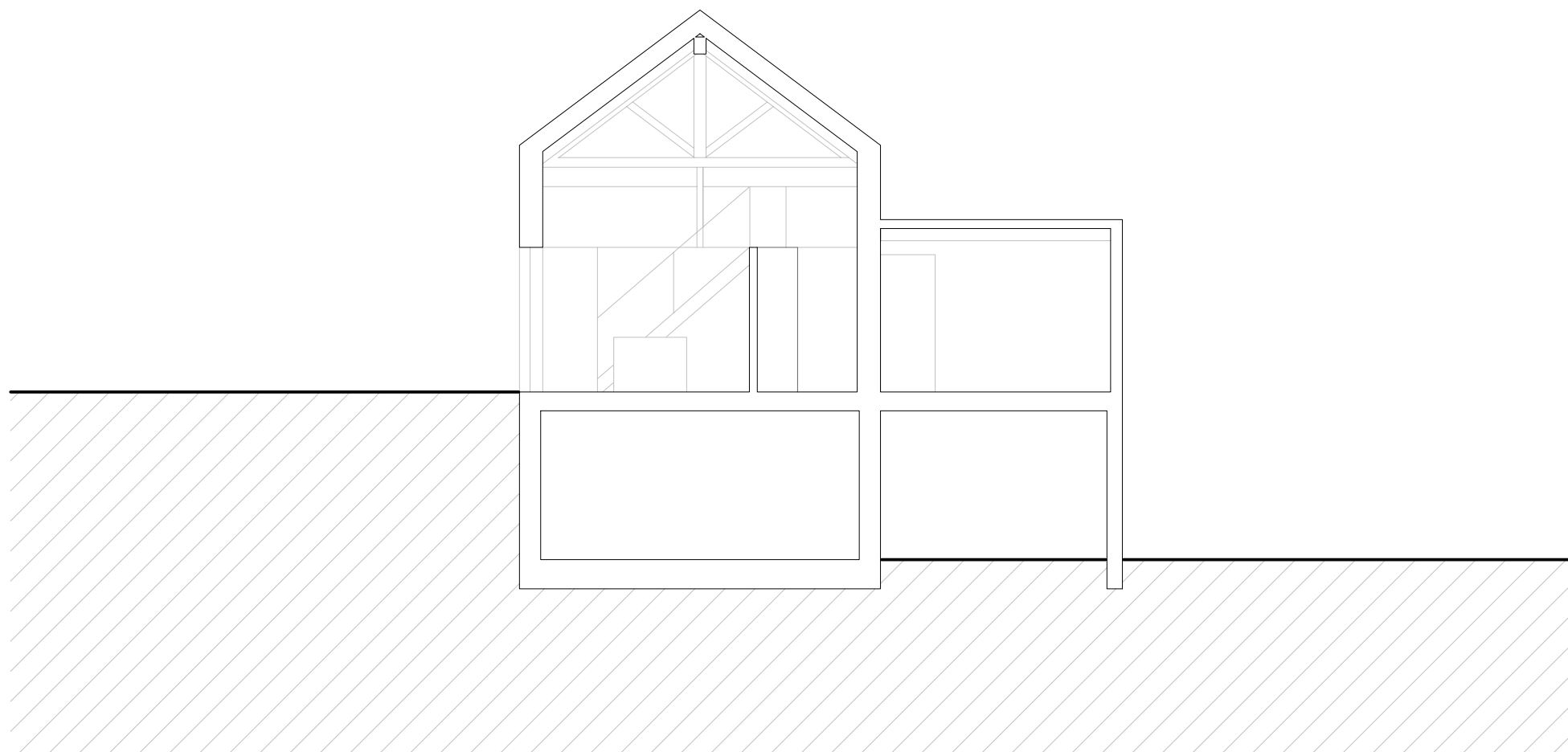
Schnitt AA 1:100
