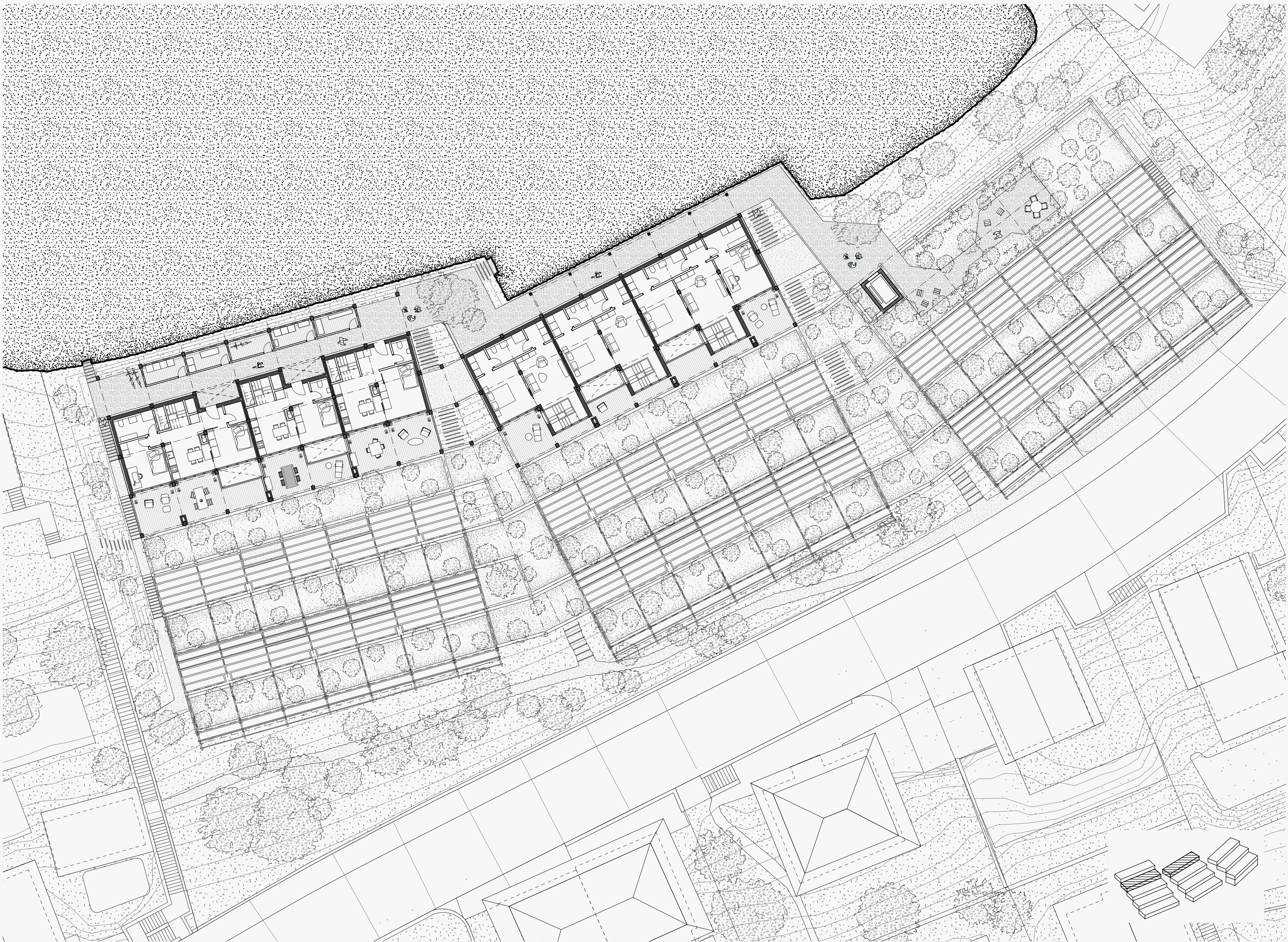
Grundriss Ebene 4 1:200
