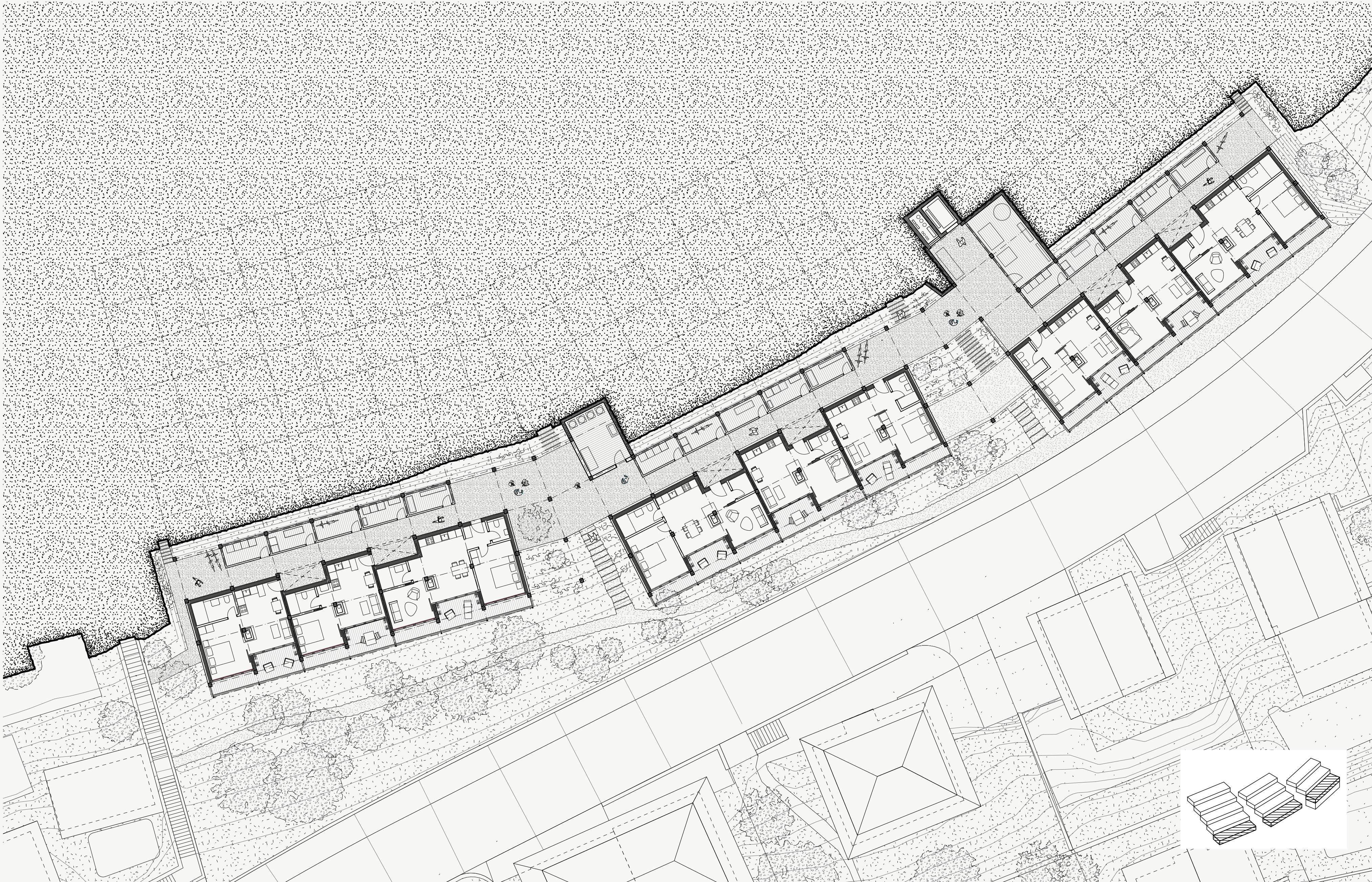
Grundriss Ebene 1 1:200
