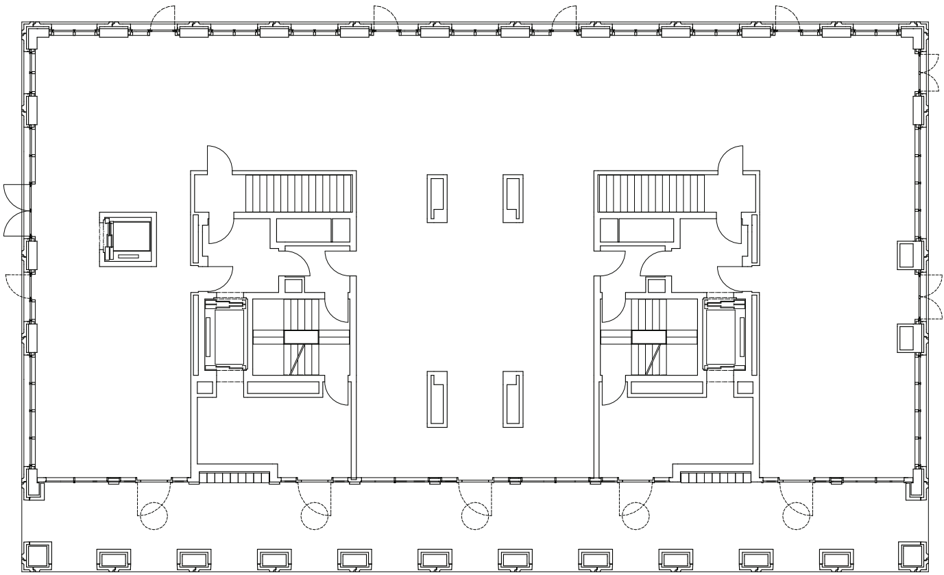
Erdgeschoss 1:200
