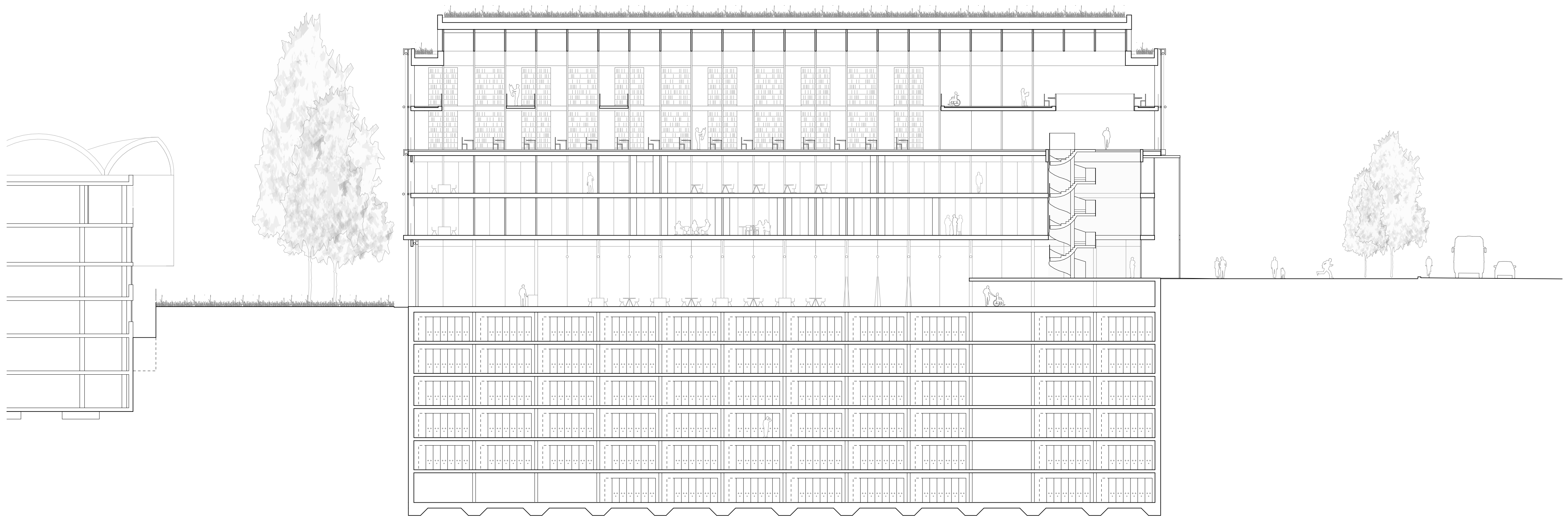
coupe longitudinale
