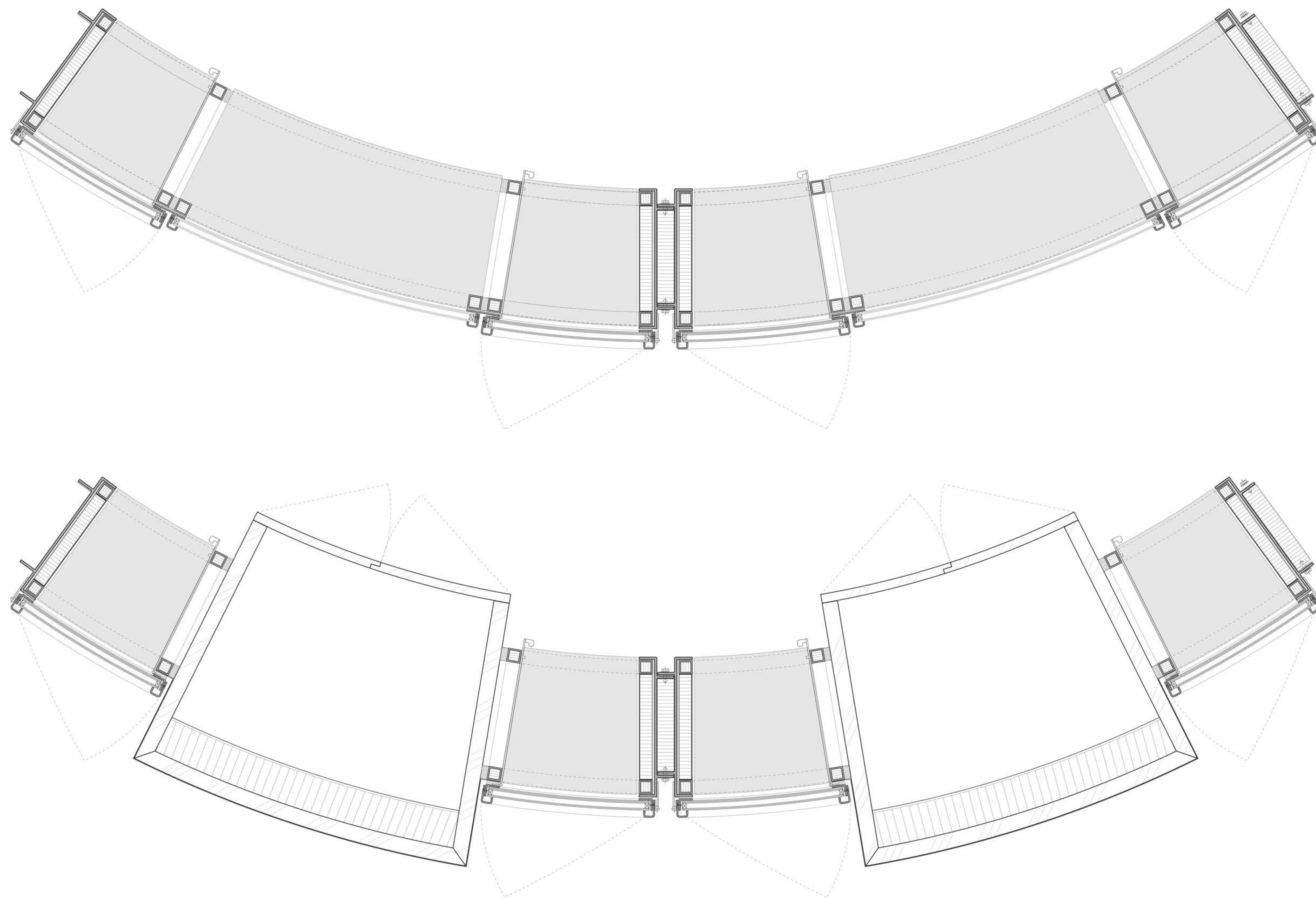
_ Fassadenmodul 1:5
