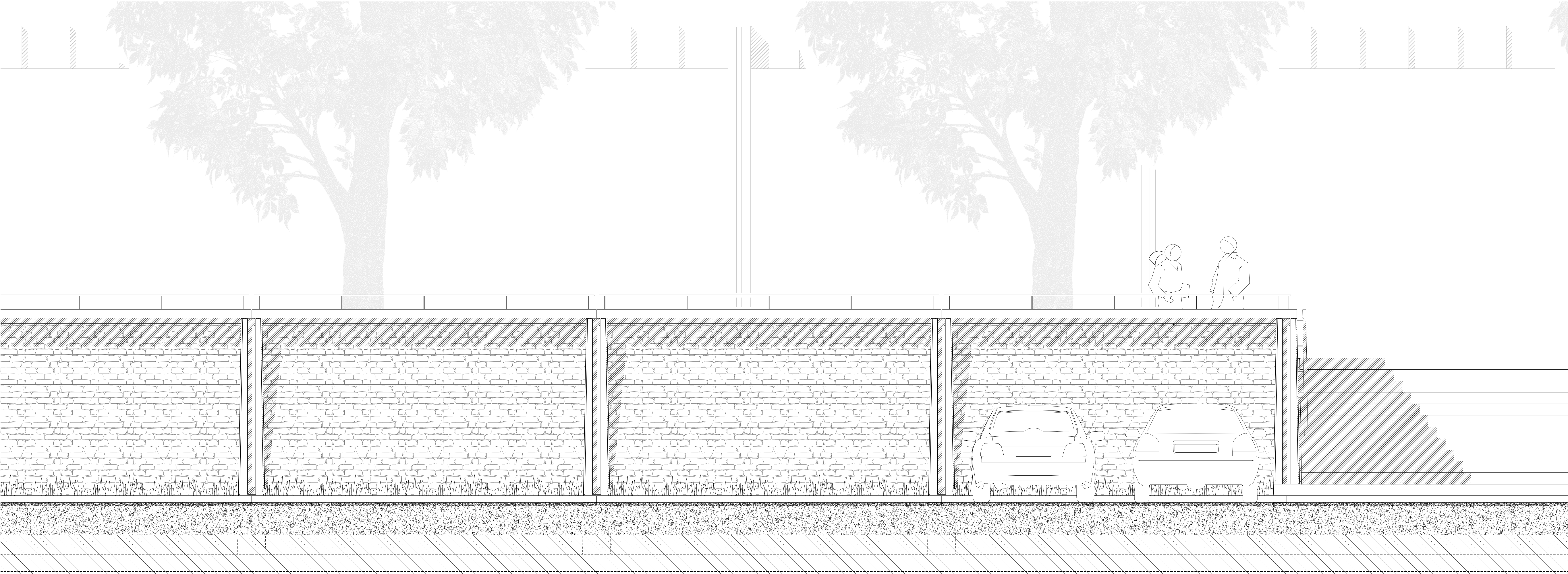
Ansicht Mauer 1_20
