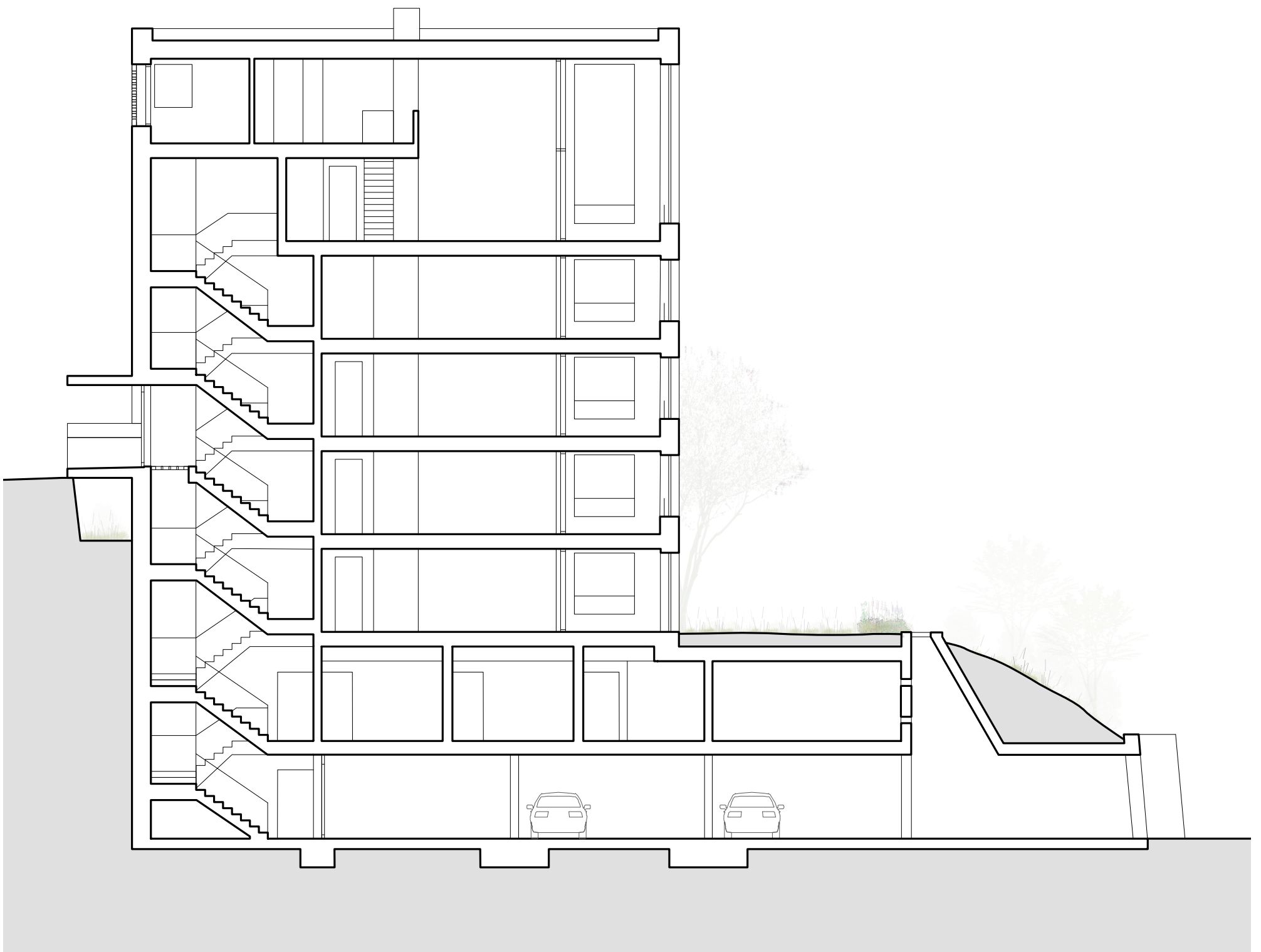
Schnitt B-B'
