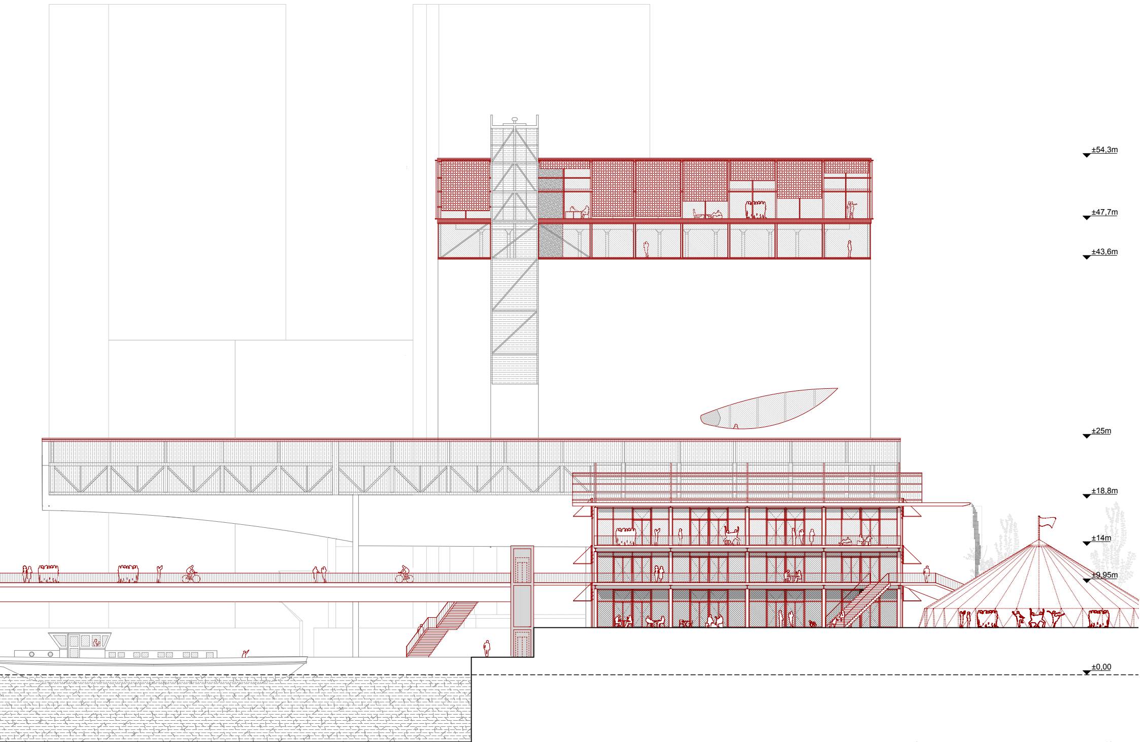
Nord Elevation
