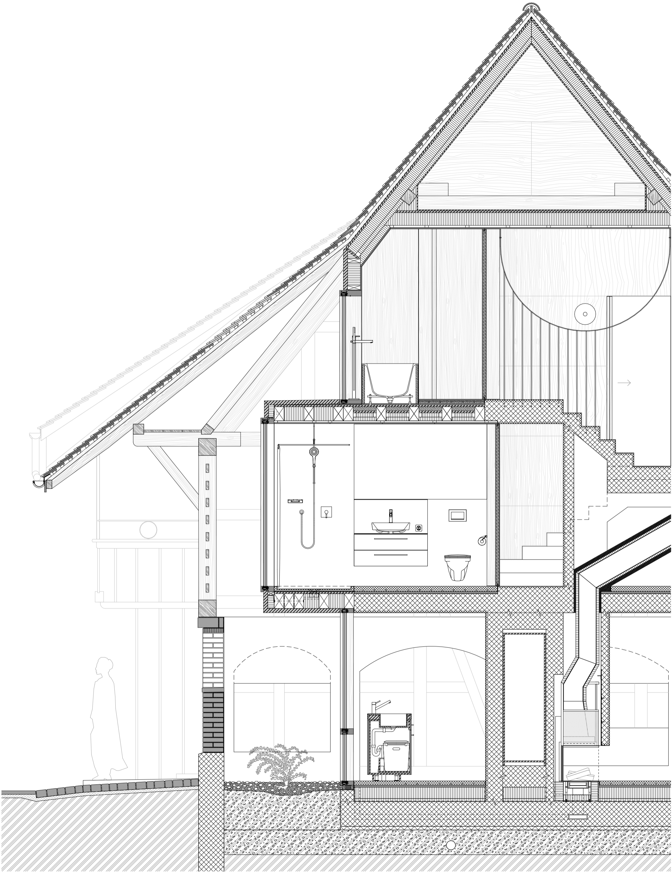
DETAILSCHNITT - HAUS IM HAUS
