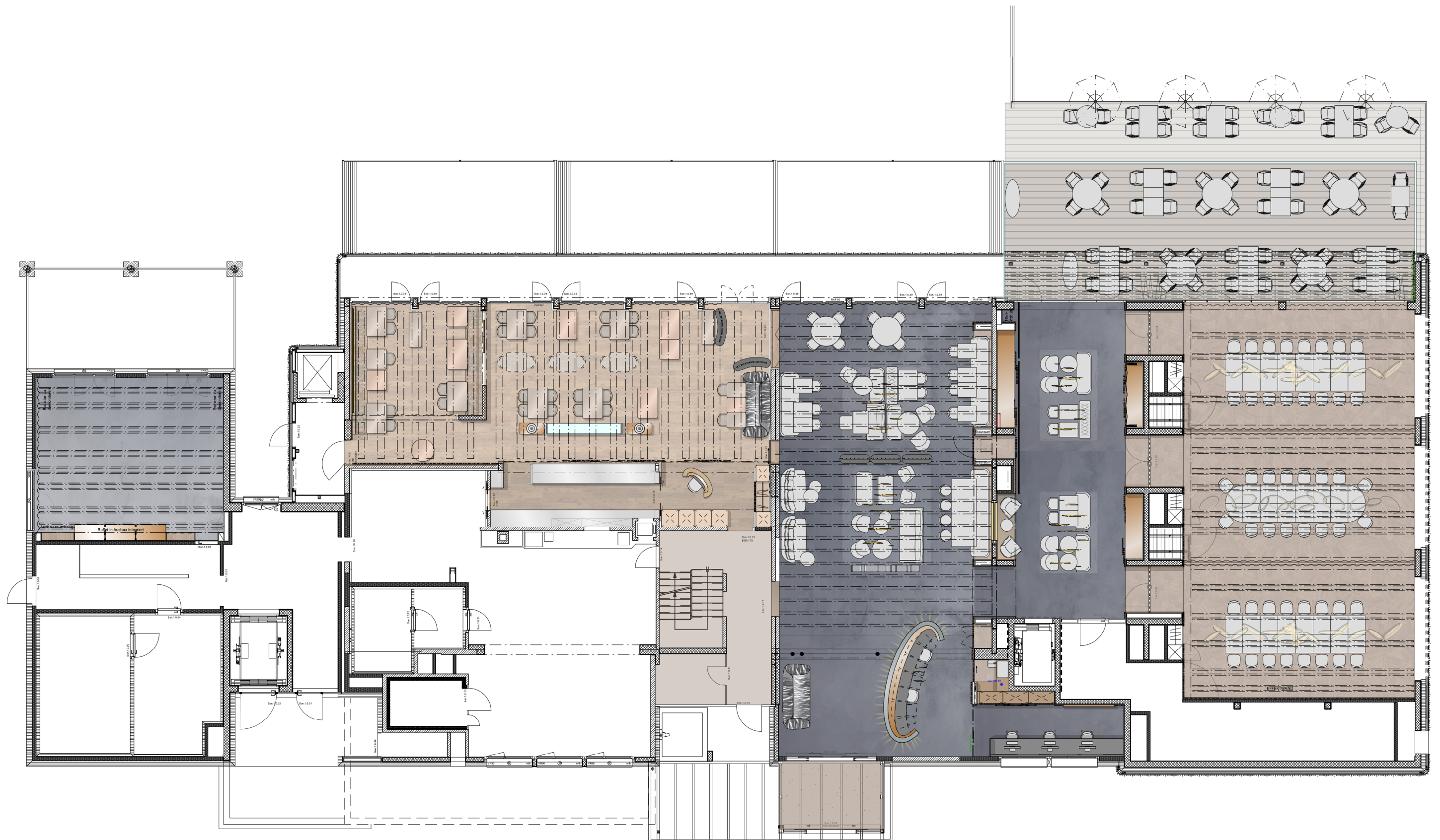
Grundriss EG | Mst. 1:150
