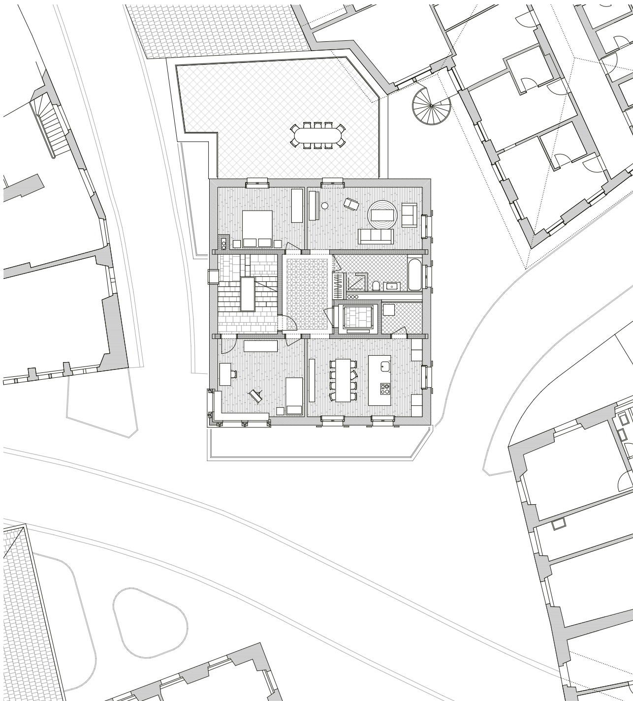
3. OBERGESCHOSS 1:200 ☉
