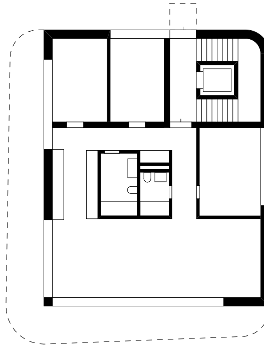
Grundriss EG
