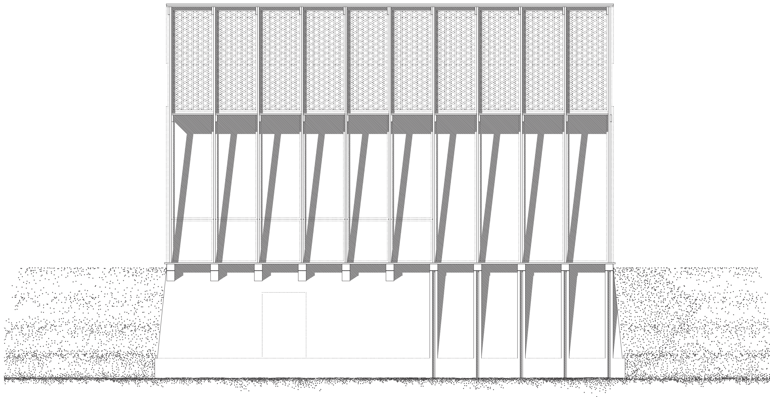
Façade est - échelle 1.50 -
