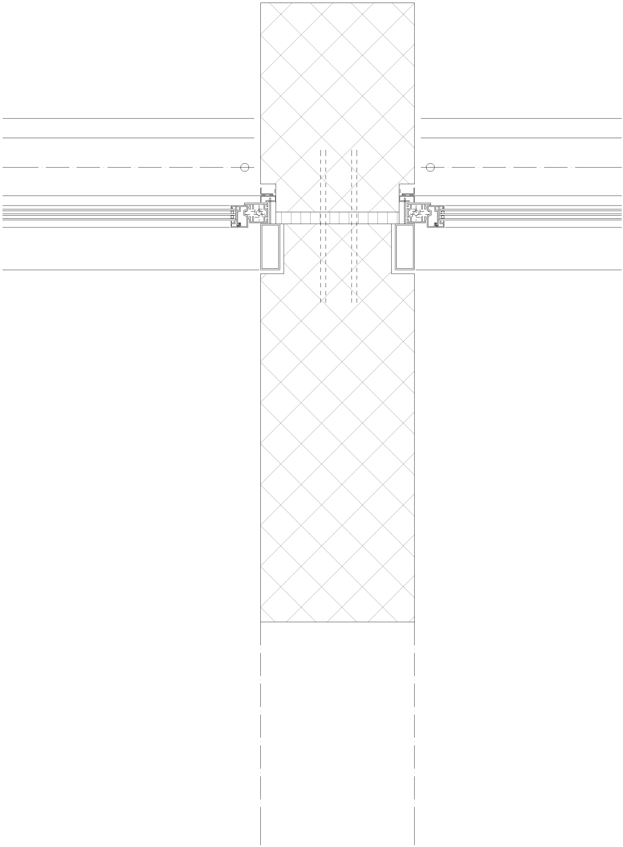
Detailschnitt Grundriss Fenster 1:10
