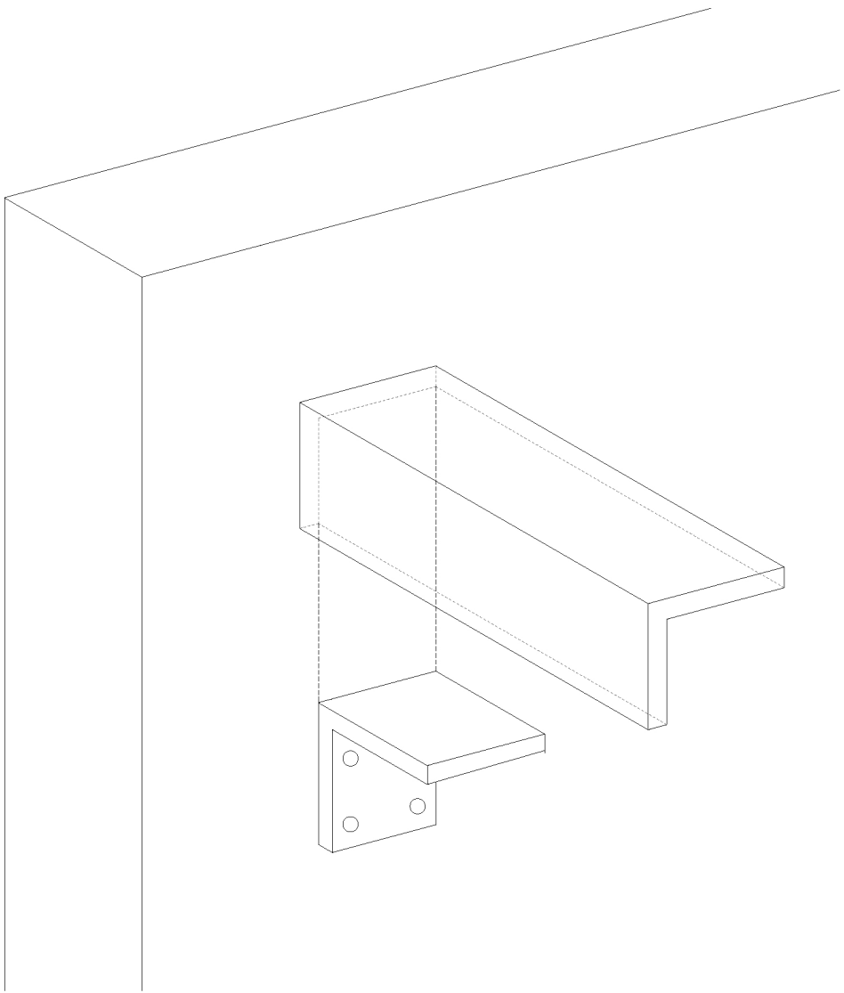
Wandmontage Winkel für Storen Axonometrie
