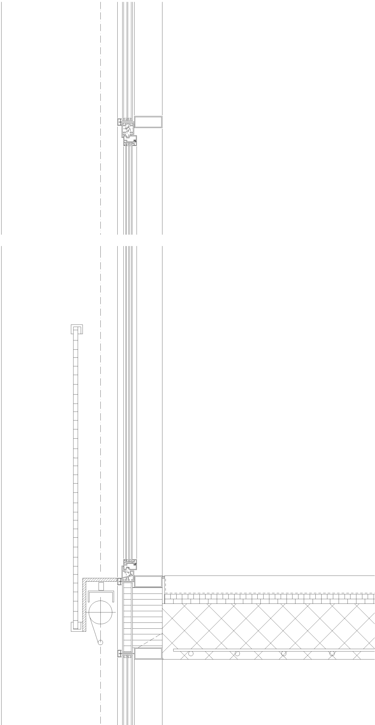
Detailschnitt Fenster 1:10
