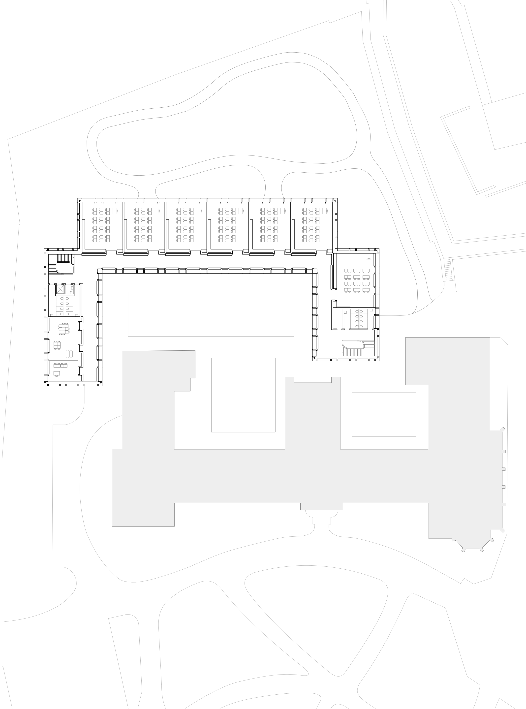
Nouvelle école du Sacré-Coeur à Estavayer-le-Lac Plan du 1er étage
