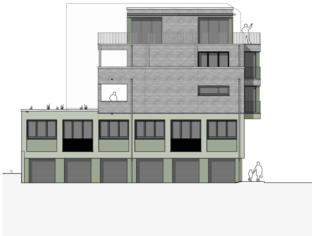
Westansicht
