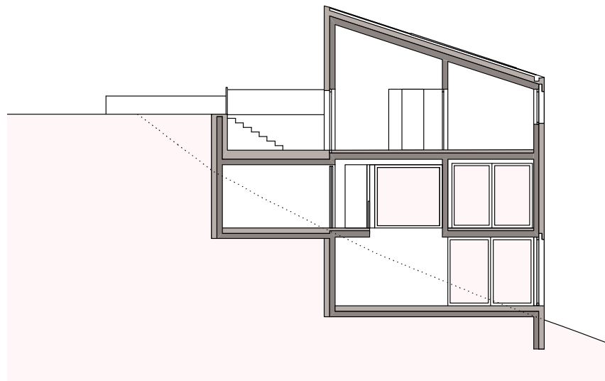
COUPE A-A
