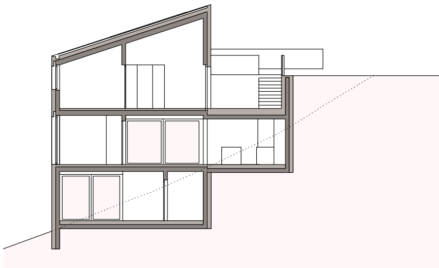
COUPE D-D
