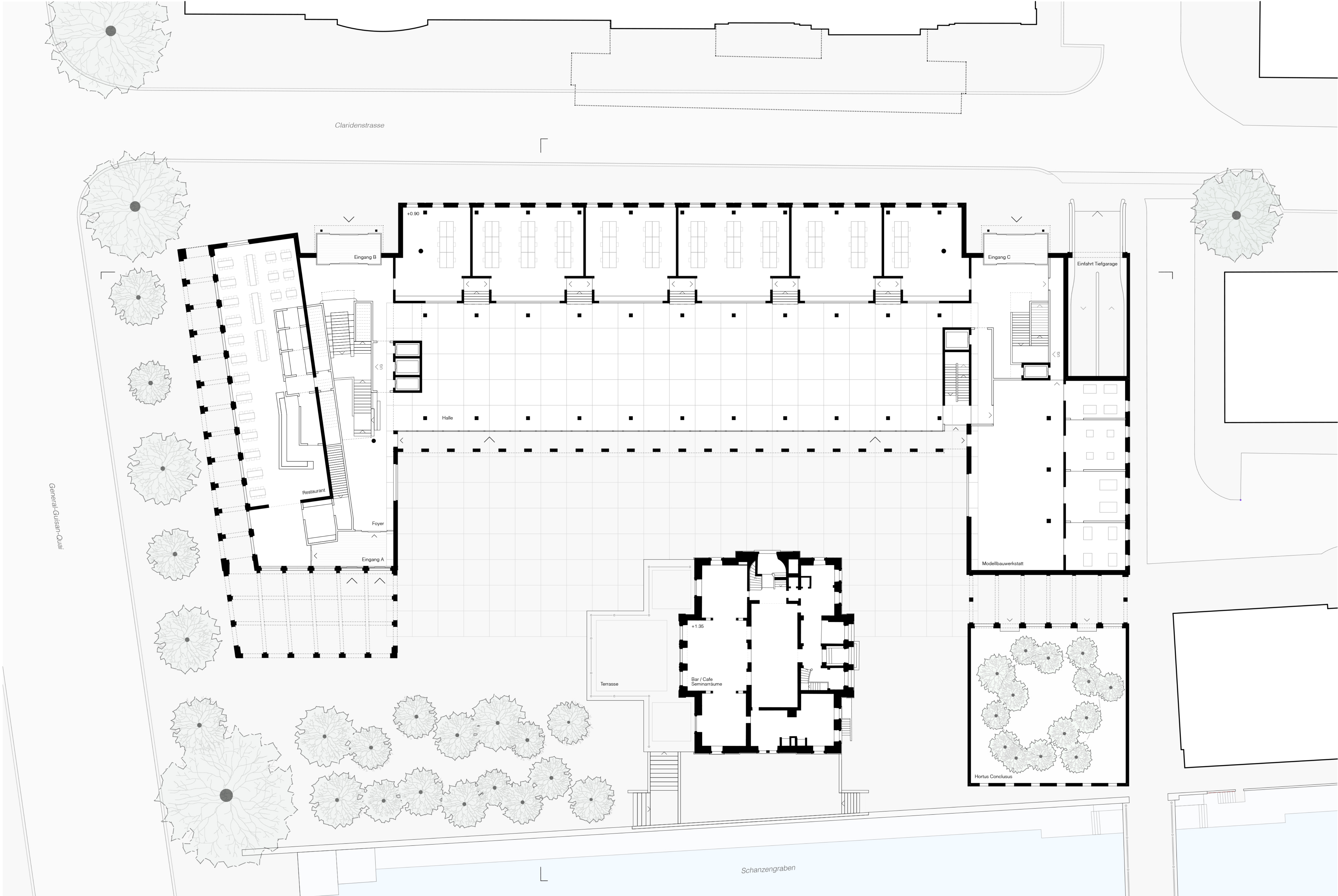
Grundriss Erdgeschoss 200
