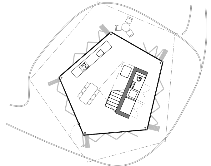
Erdgeschoss 1:200
