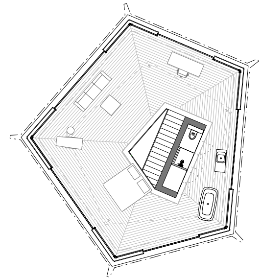
Obergeschoss 1:200
