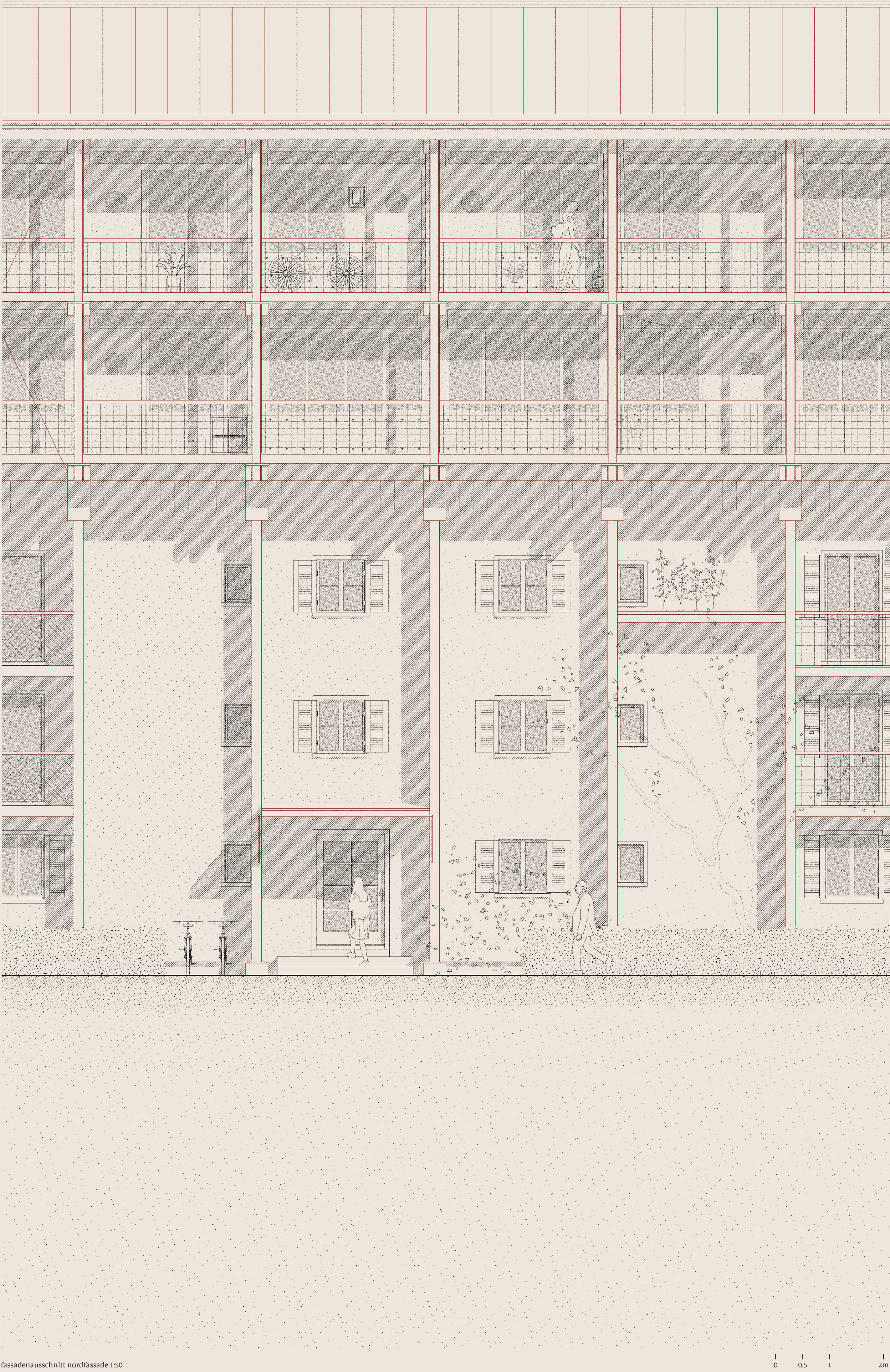
fassadenausschnitt nordfassade 1:50
