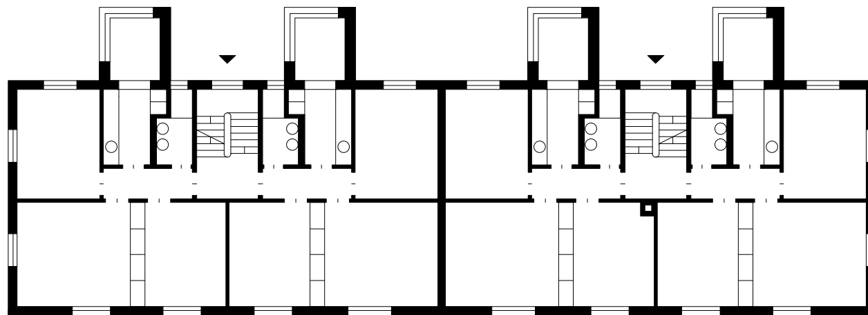
GRUNDRISS EG
