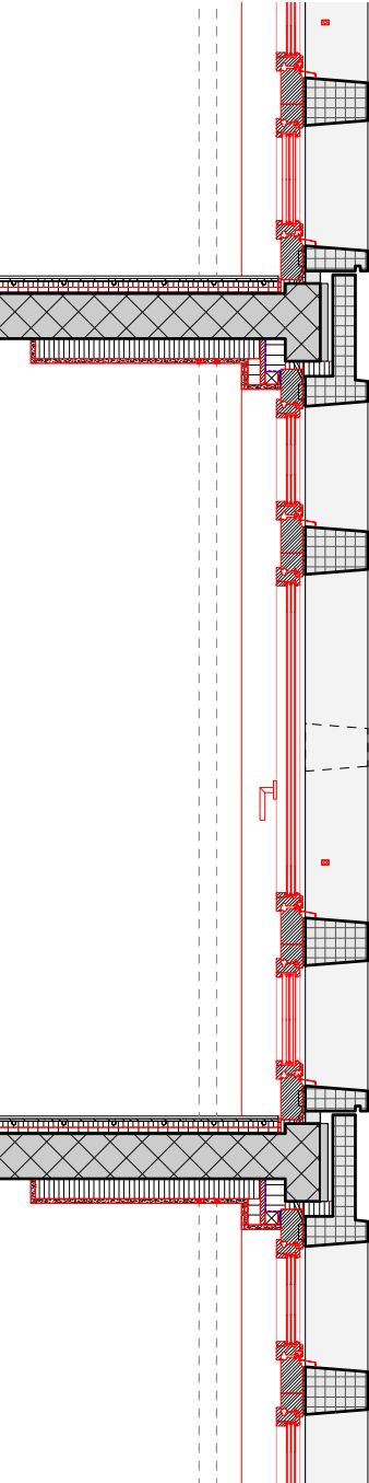
SCHNITT Mst. 1:33
