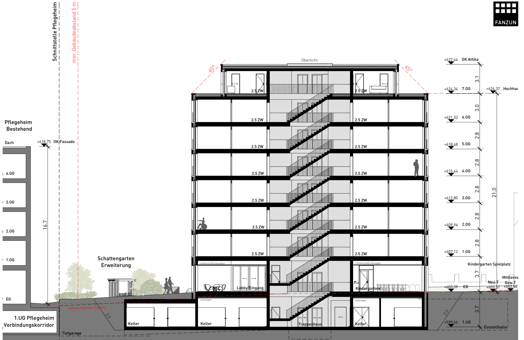
Haus am Mühlbach, Alterssiedlung Bodmer, Chur Baudokumentation | Längsschnitt AA
