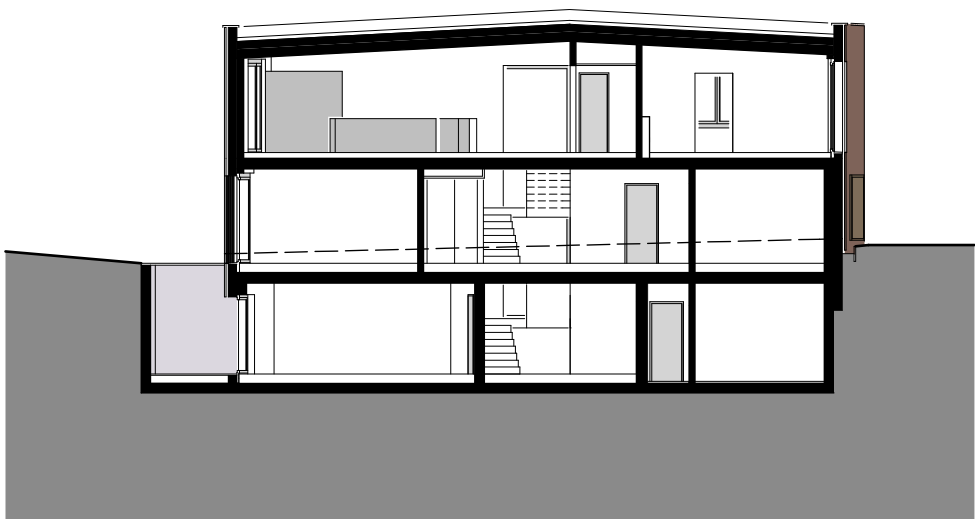
EFH Längsschnitt
