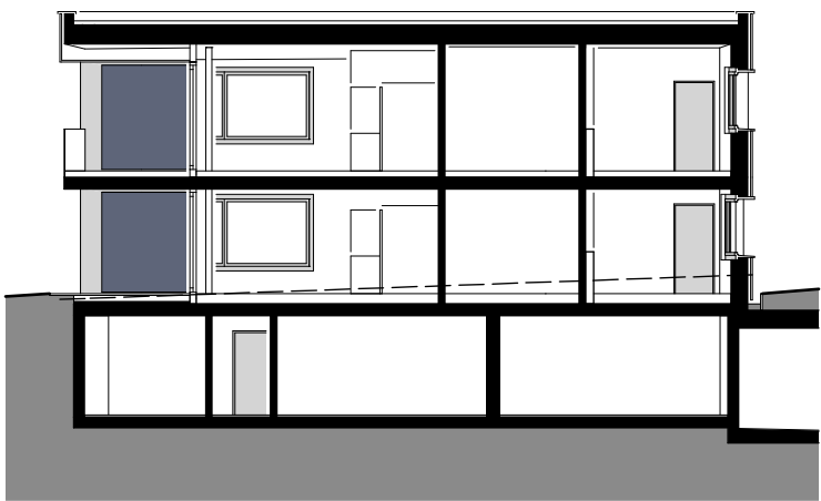
MFH Querschnitt
