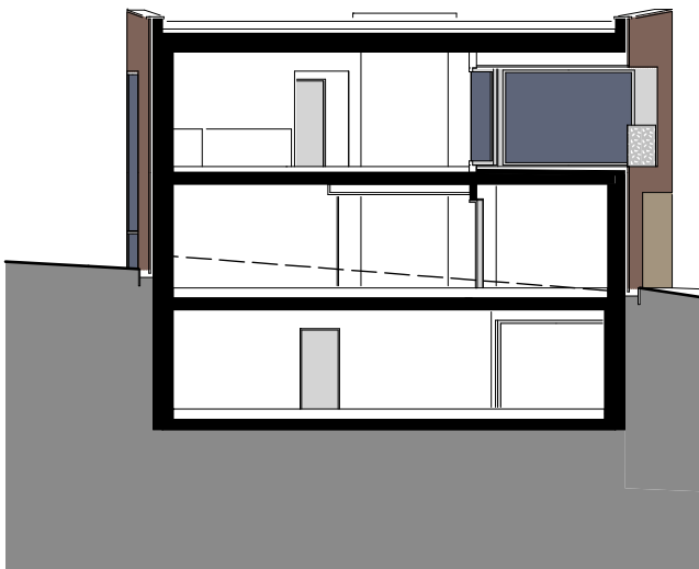
EFH Querschnitt
