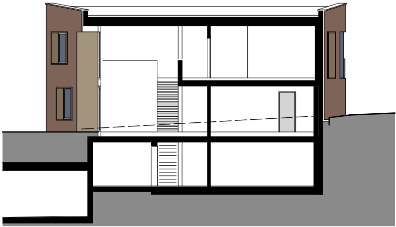
DEFH Querschnitt
