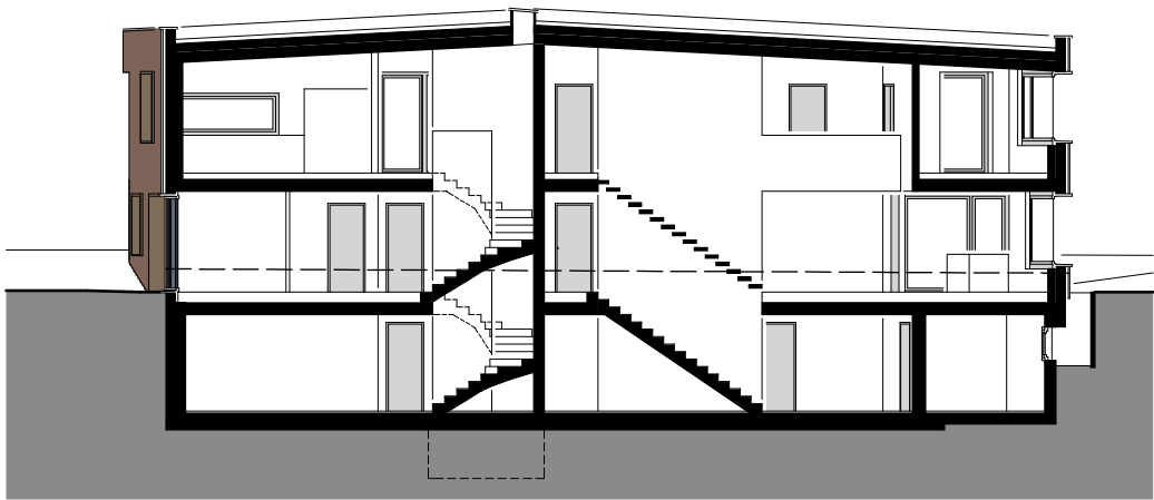
DEFH Längsschnitt
