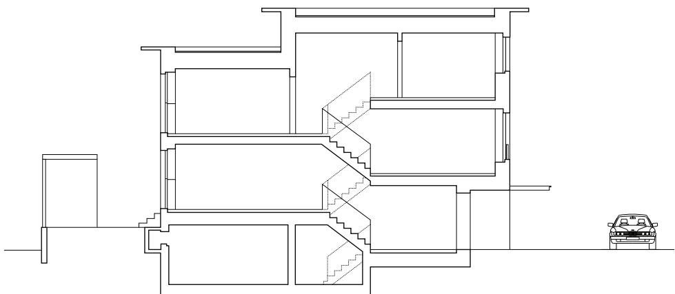
Schnitt
