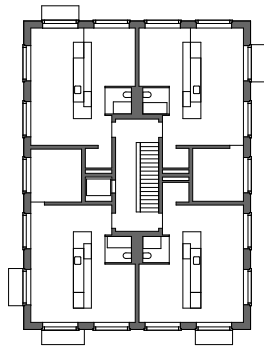
Regelgeschoss, Haus C
