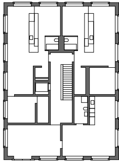
Grundriss Erdgeschoss, Haus C
