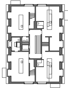
1. Dachgeschoss, Haus C
