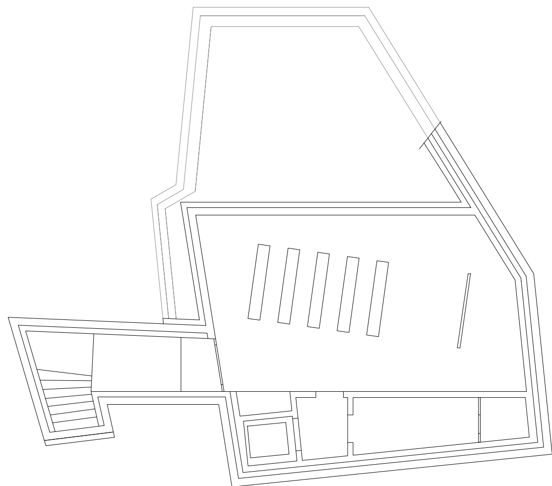
plan sous-sol
