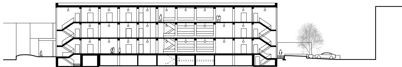
Längsschnitt 1:500
