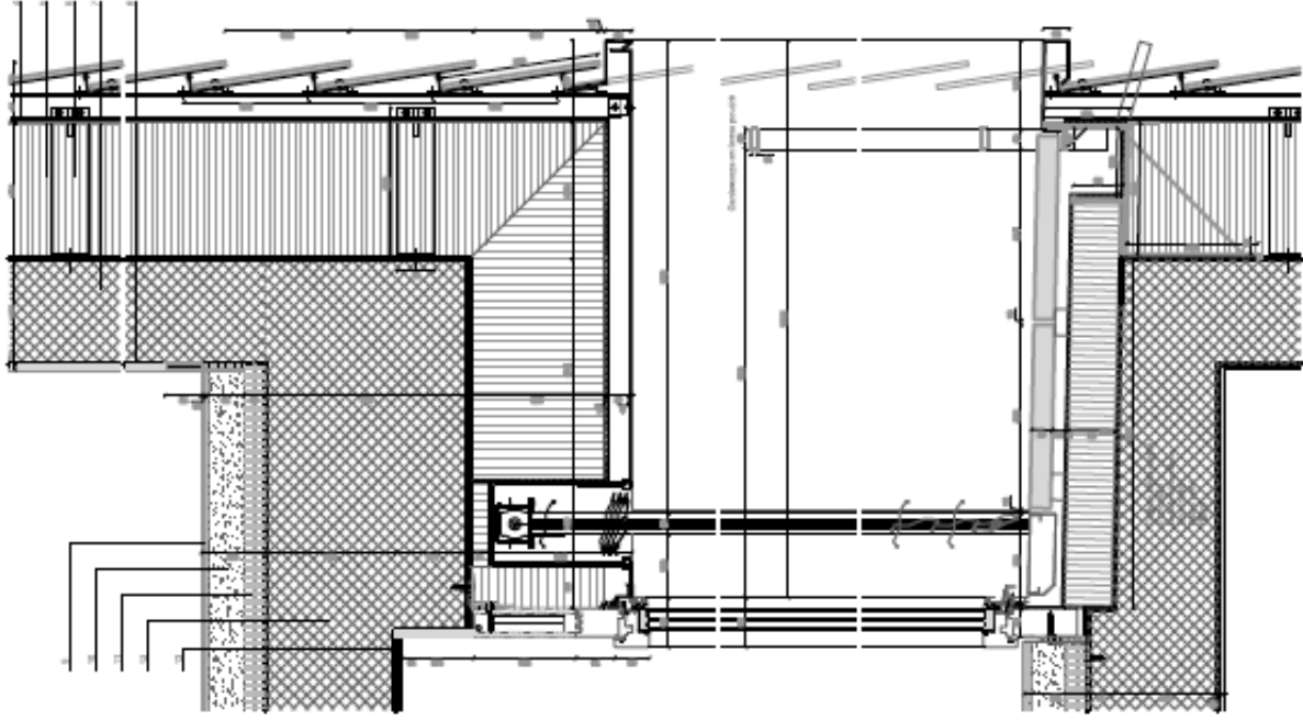
DETAIL CONSTRUCTIF éch. 1/40
