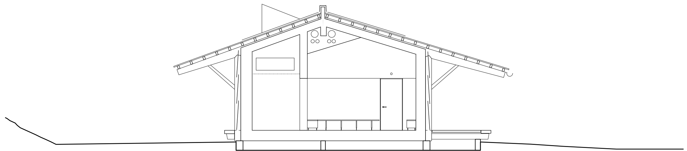
Coupe A
