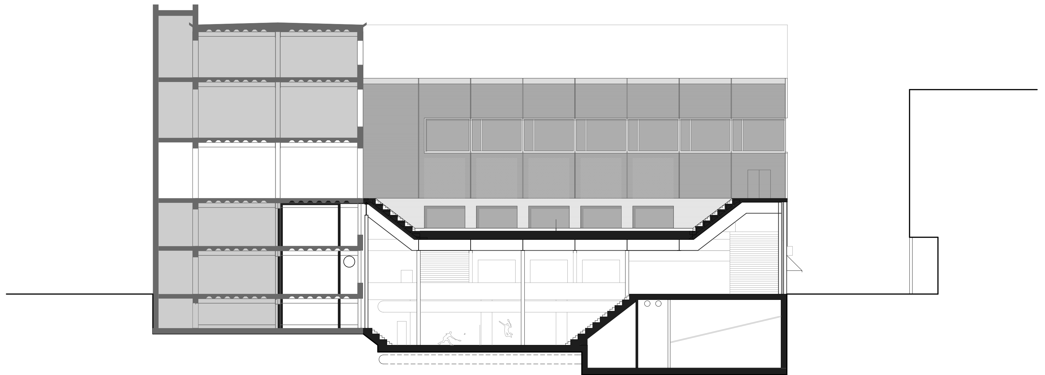
Schnitt C-C 1:200
