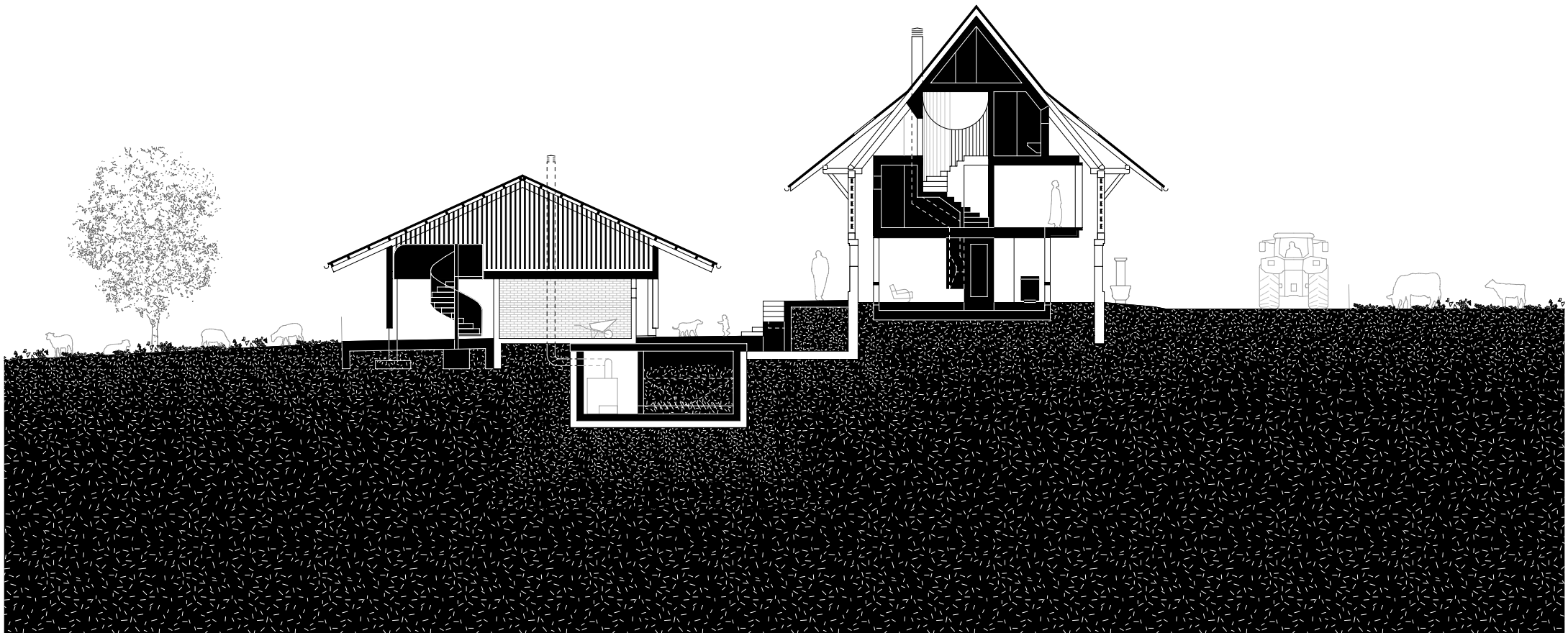
QUERSCHNITT - HAUS IM HAUS / NEBENGEBÄUDE
