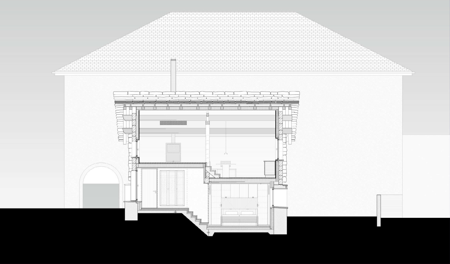
al Sezione camera e vestibolo si Viste camera con bagno
