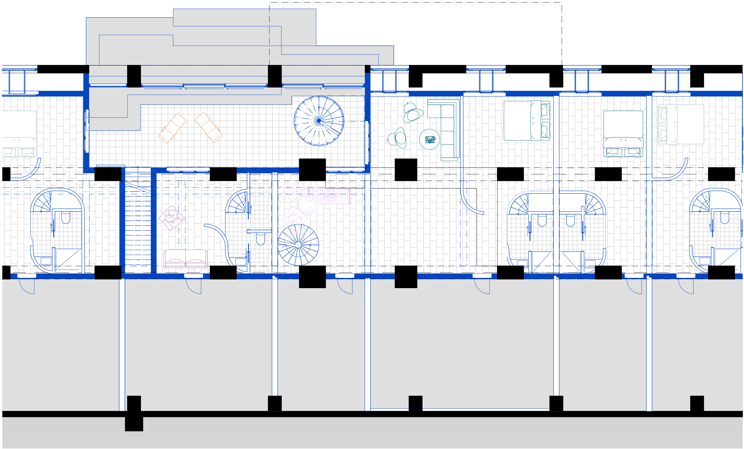
Grundriss Untergeschoss | 1:100
