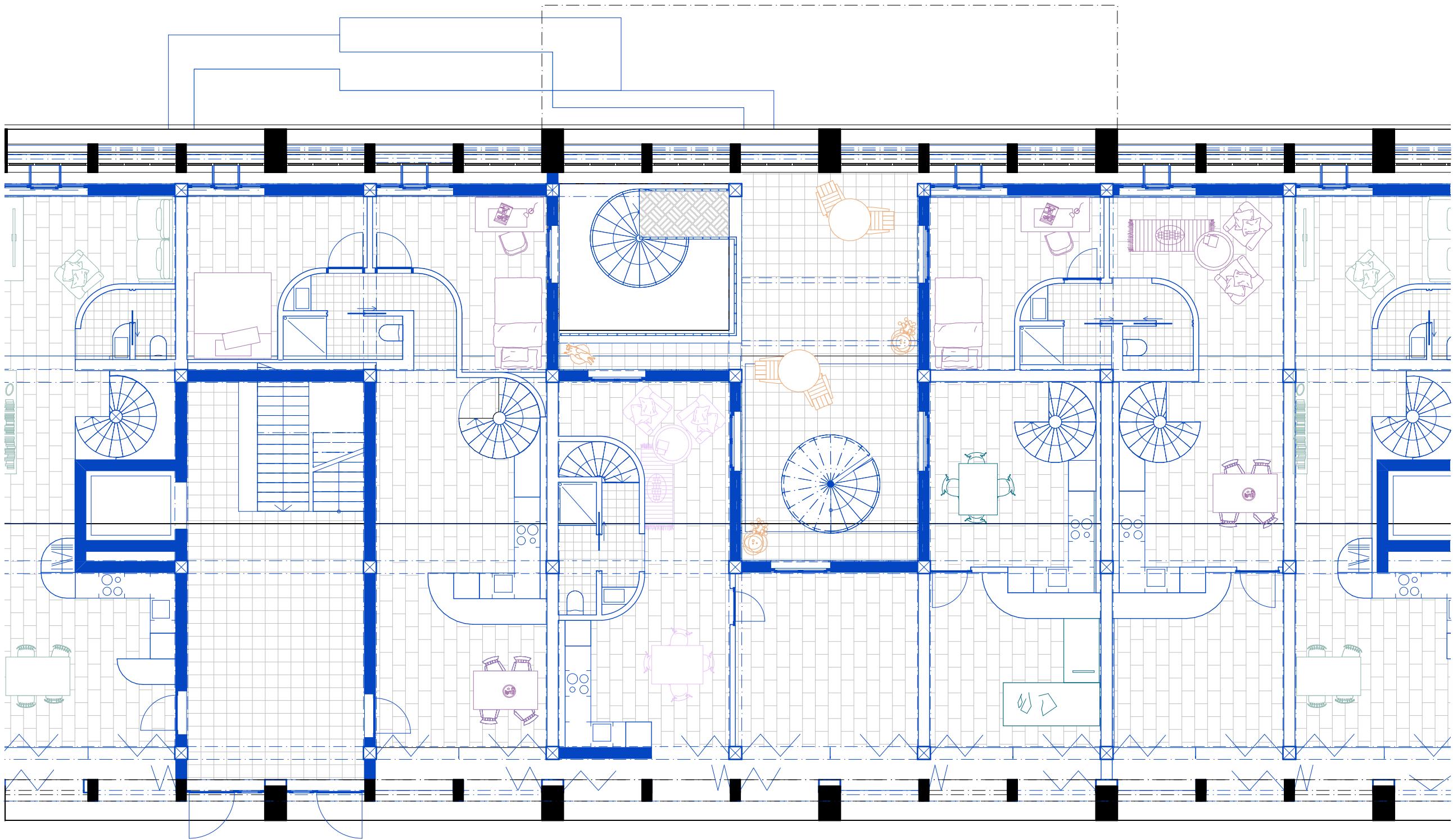
Grundriss Erdgeschoss | 1:100
