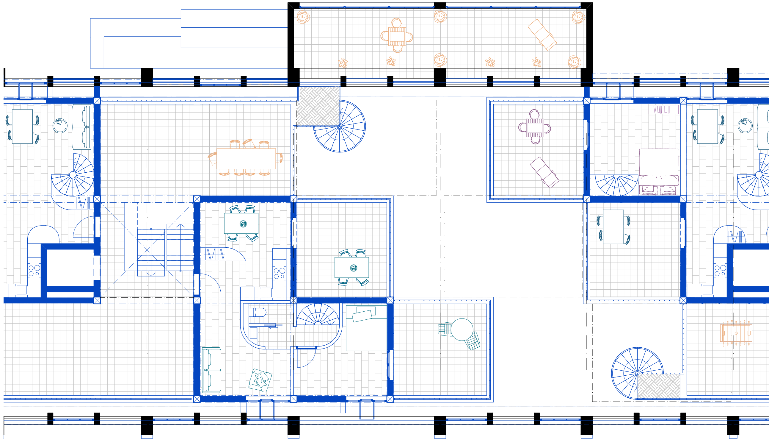
Grundriss 2.Obergeschoss | 1:100
