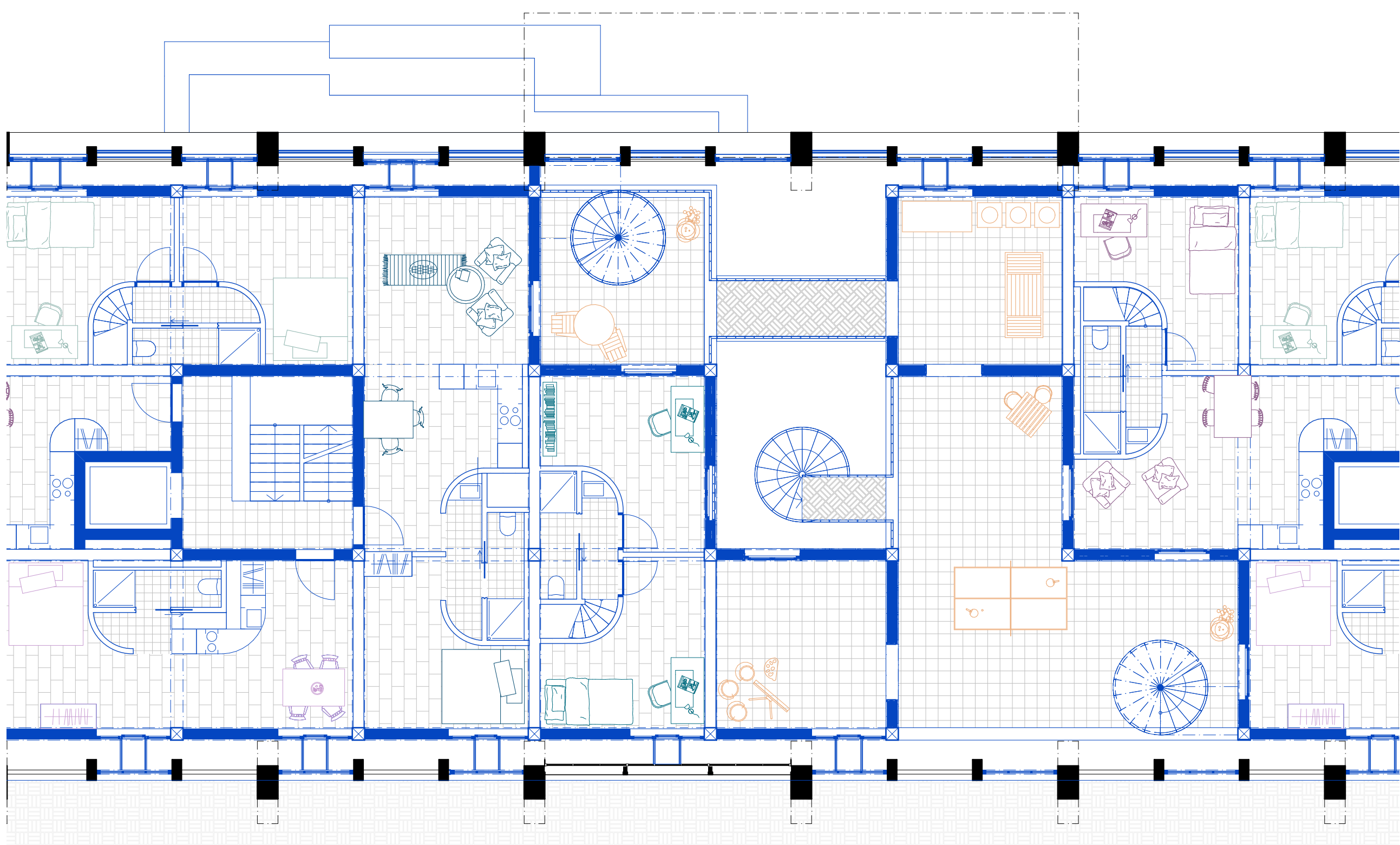
Grundriss 1.Obergeschoss | 1:100
