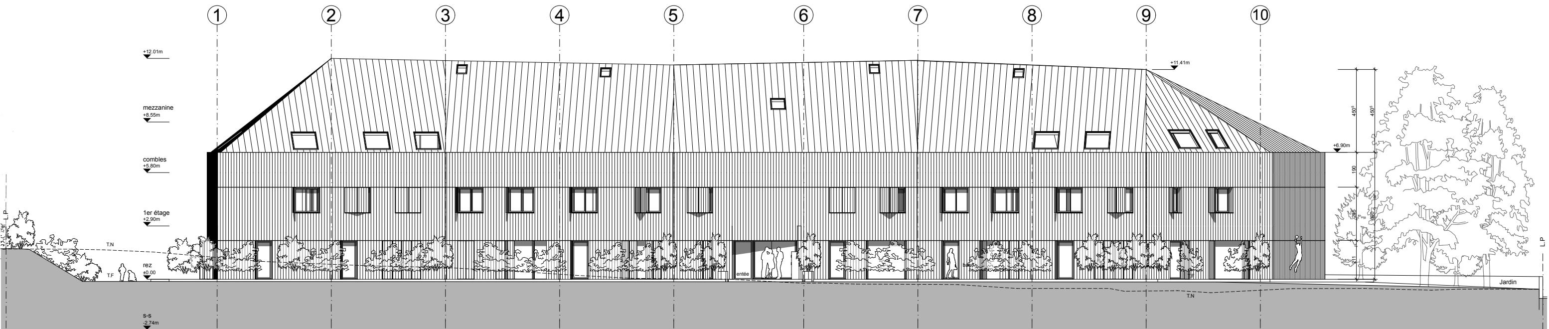
FACADE EST - Chemin des Vernaz
