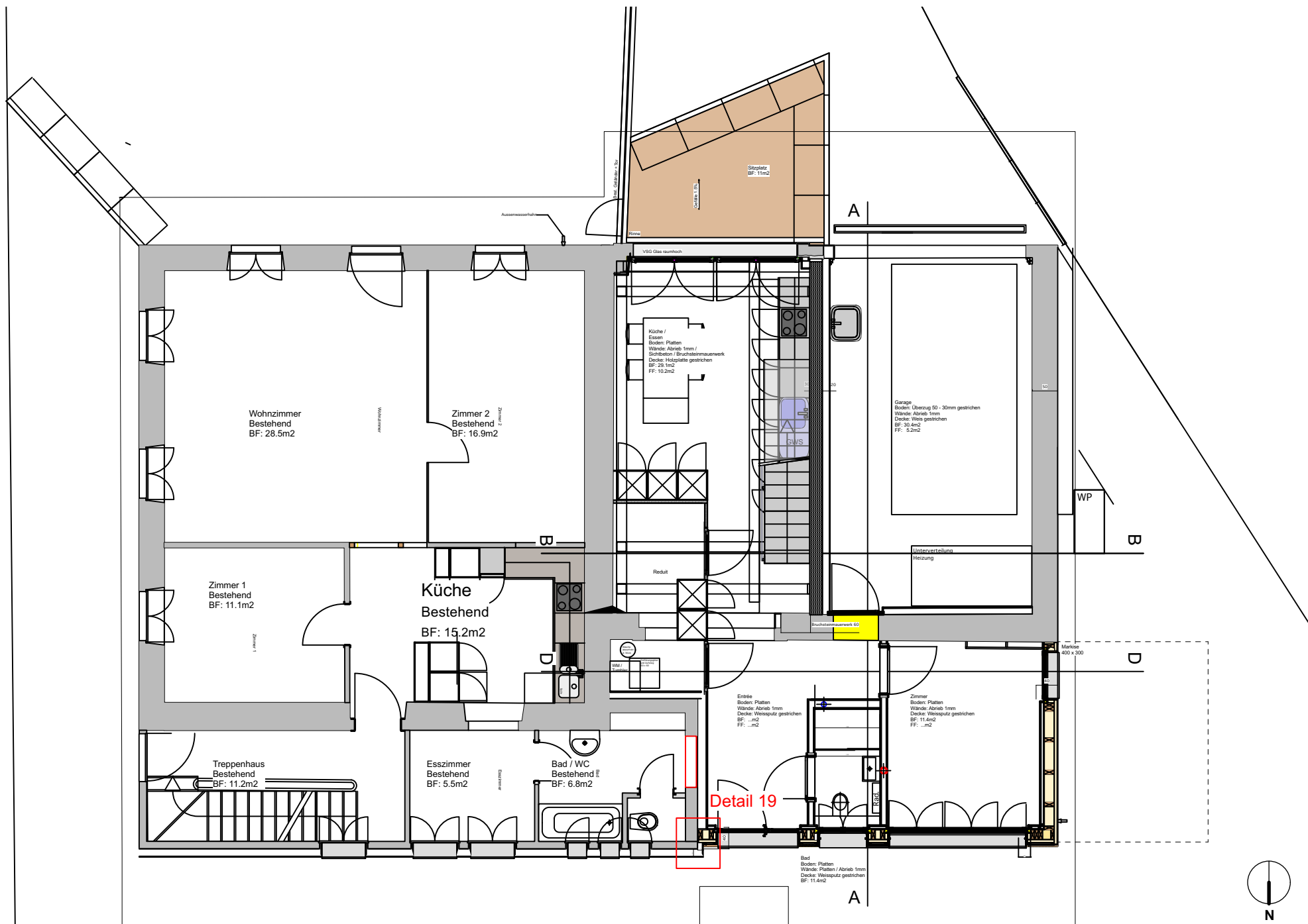
Erdgeschoss 1:100
