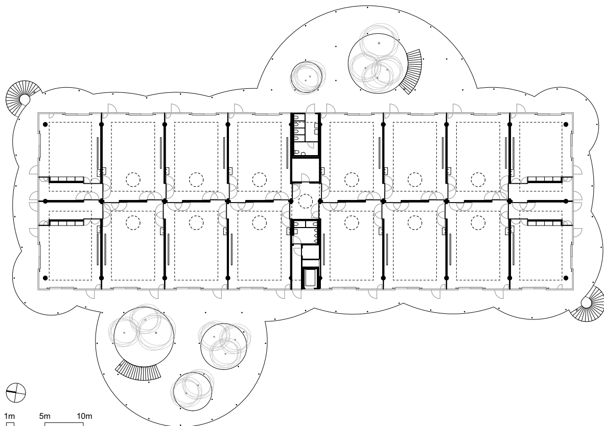
Grundriss 2. OG 1:500
