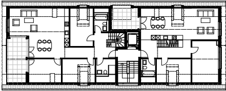
1. Dachgeschoss Haus D | Étage sous-toiture maison D
