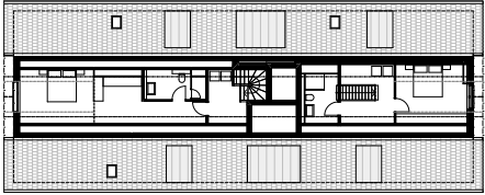
2. Dachgeschoss Haus D | Combles maison D
