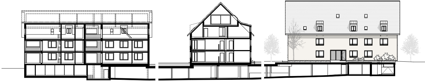
Schnitt | Coupe
