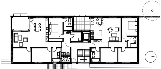
Erdgeschoss Haus D | Rez-de-chaussée maison D
