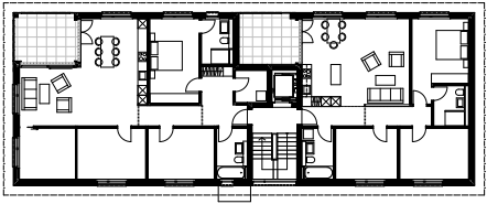
Obergeschoss Haus D | Étage maison D
