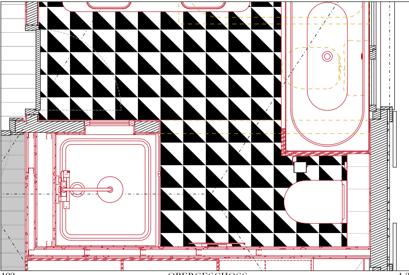
102 OBERGESCHOSS 1:33
