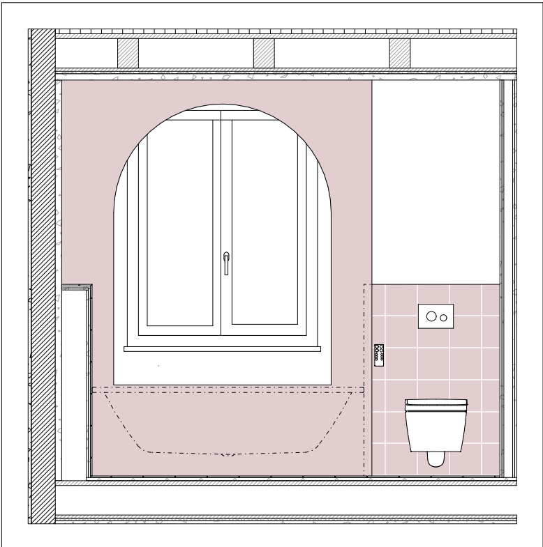
426_1A HAUPTBAD 1:33
