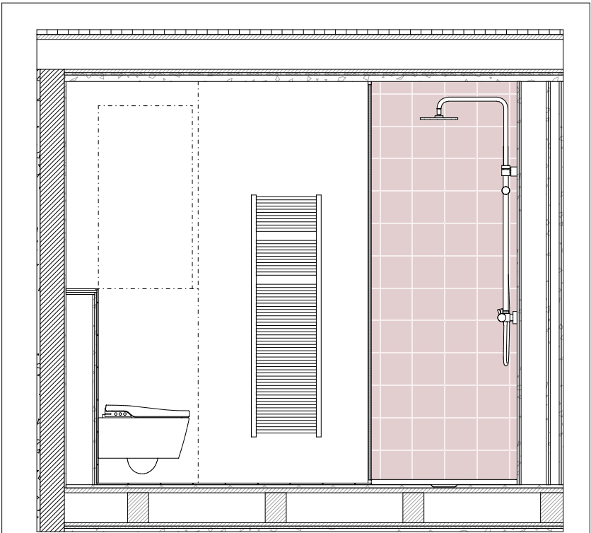
426_1A HAUPTBAD 1:33
