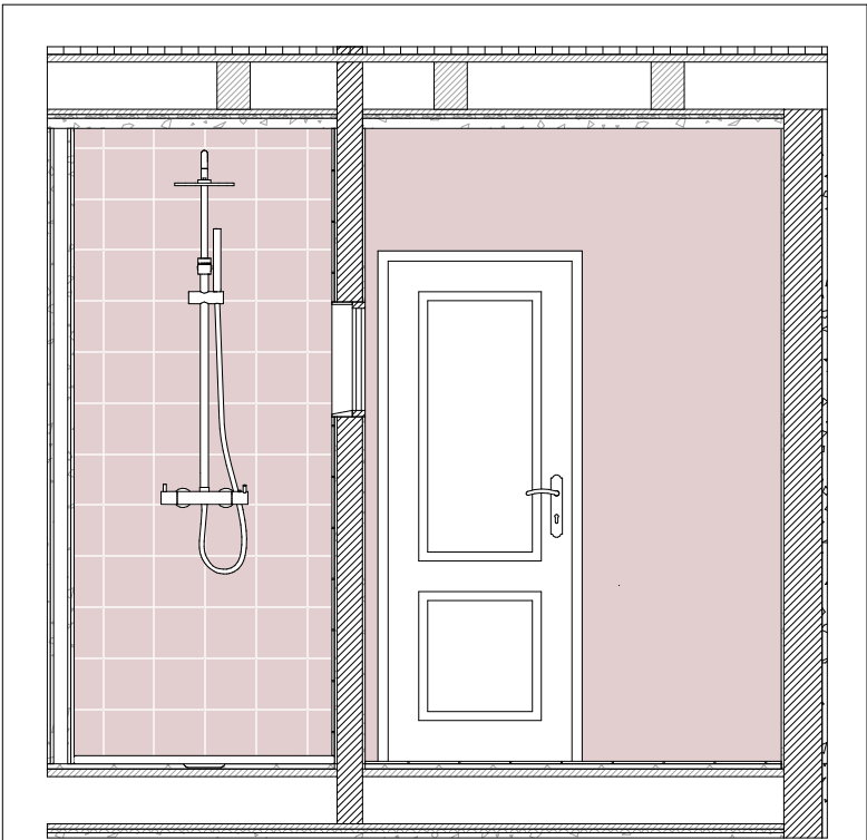
426_1A HAUPTBAD 1:33
