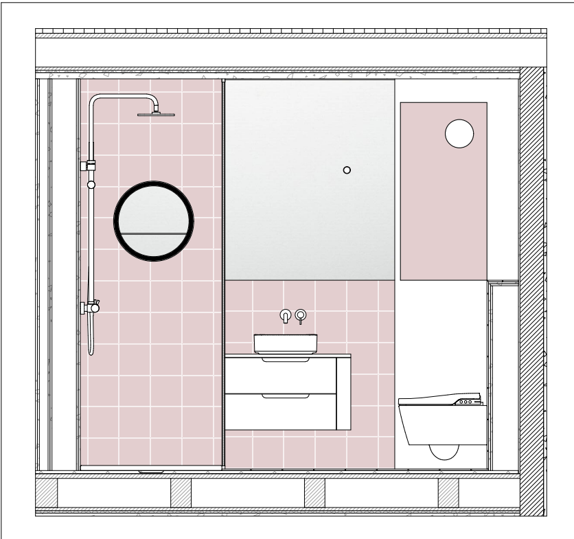
426_1A HAUPTBAD 1:33
