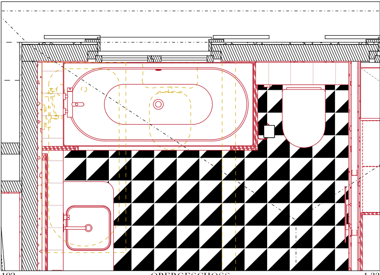
102 OBERGESCHOSS 1:33
