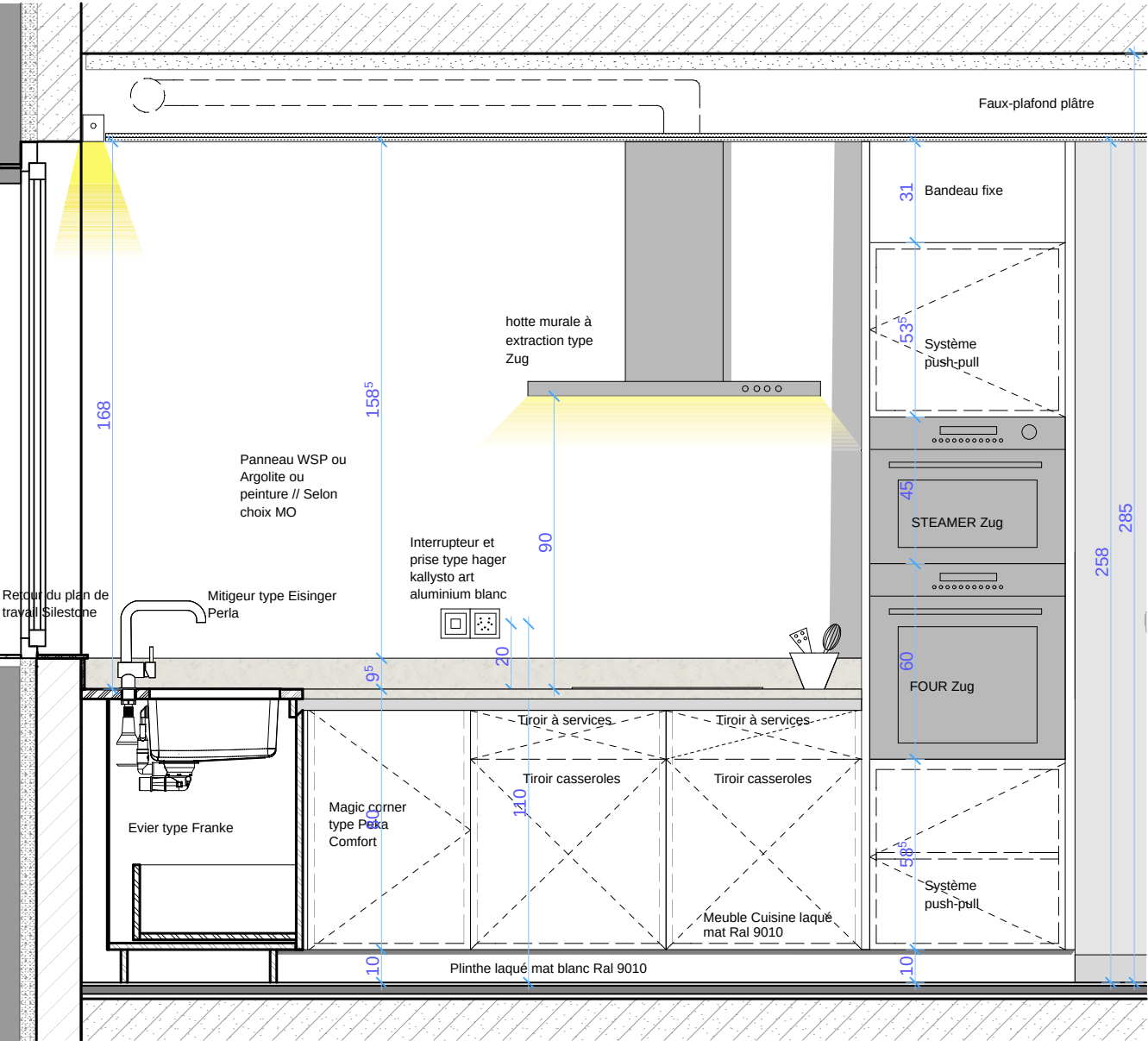
Coupe A-A
