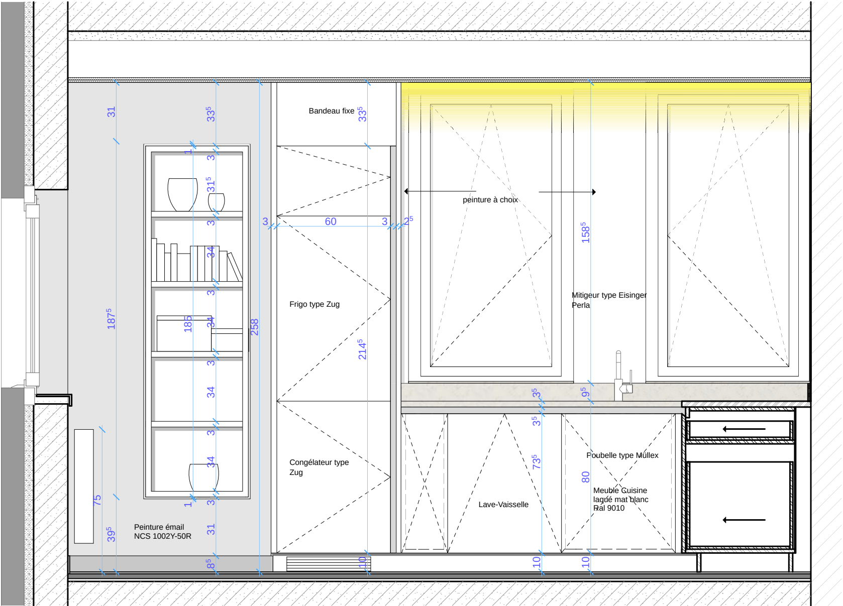
Coupe B-B
