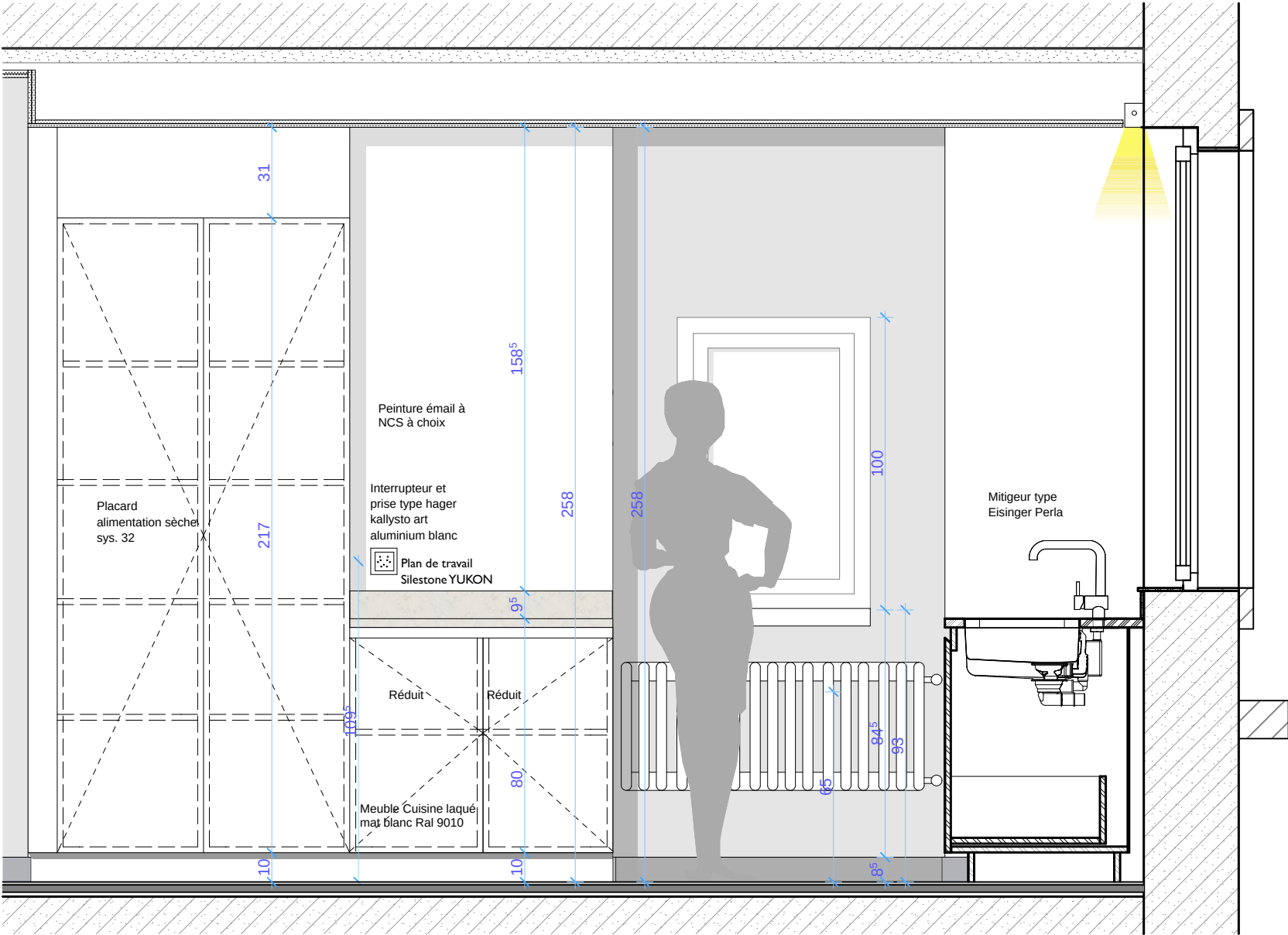
Coupe C-C
