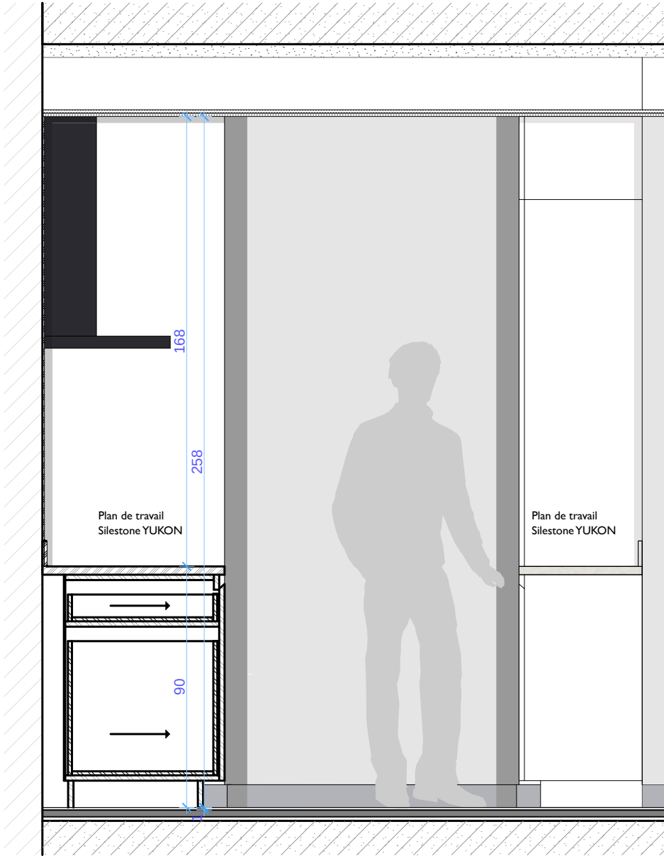
Coupe D-D
