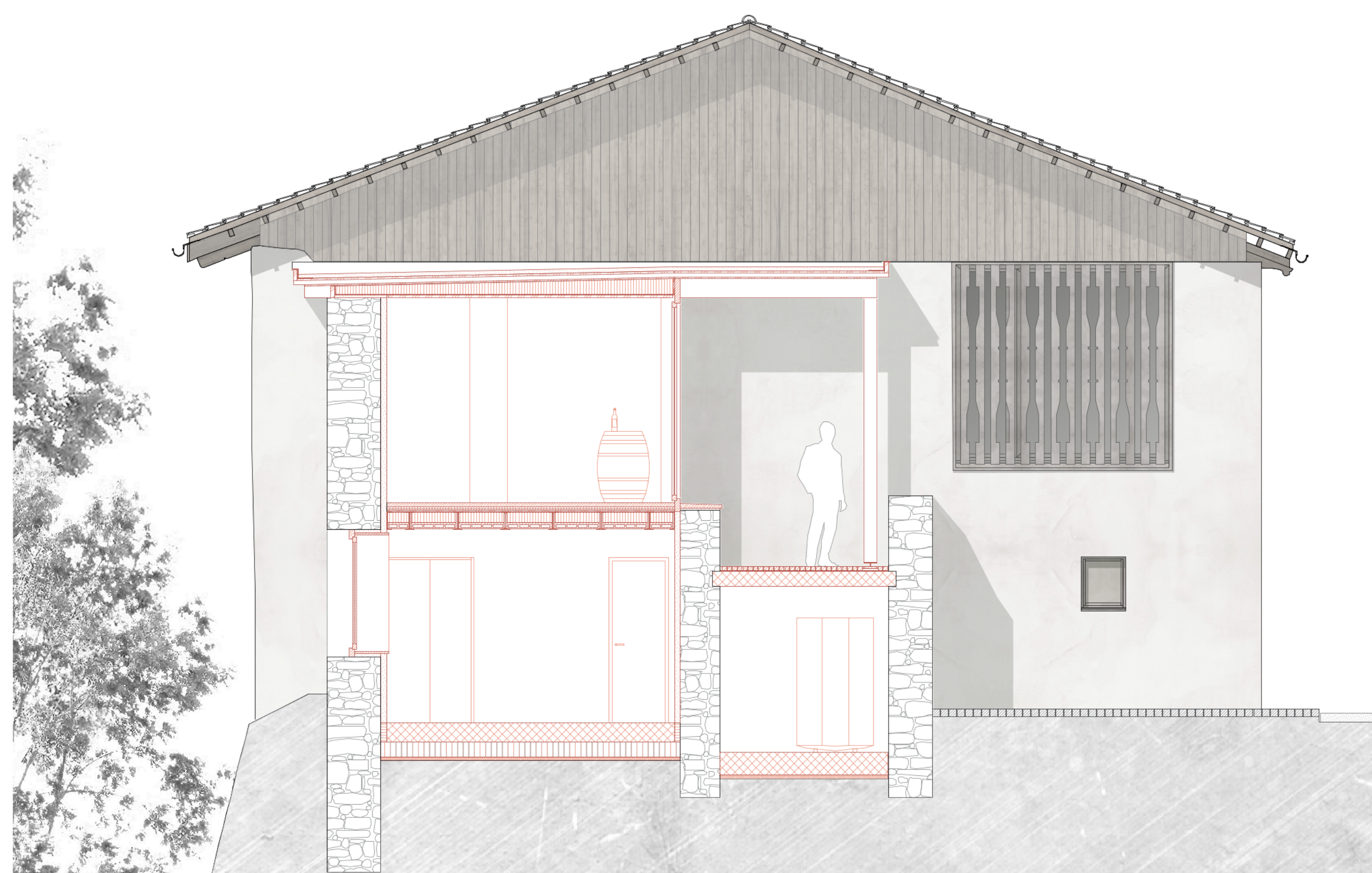
LÄNGSSCHNITT
