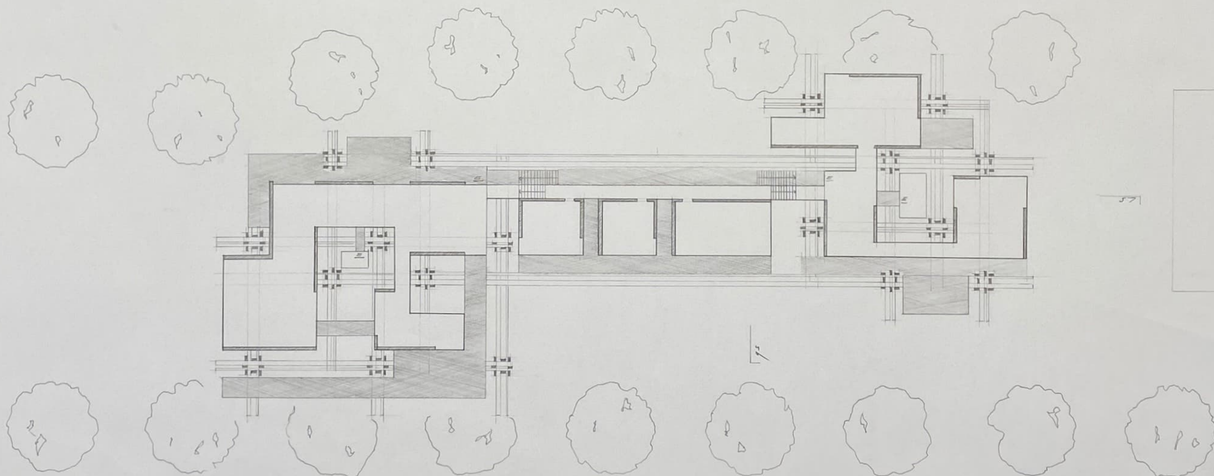
Grundriss 1.06, Mst. 1:200 Kunze, 1981
