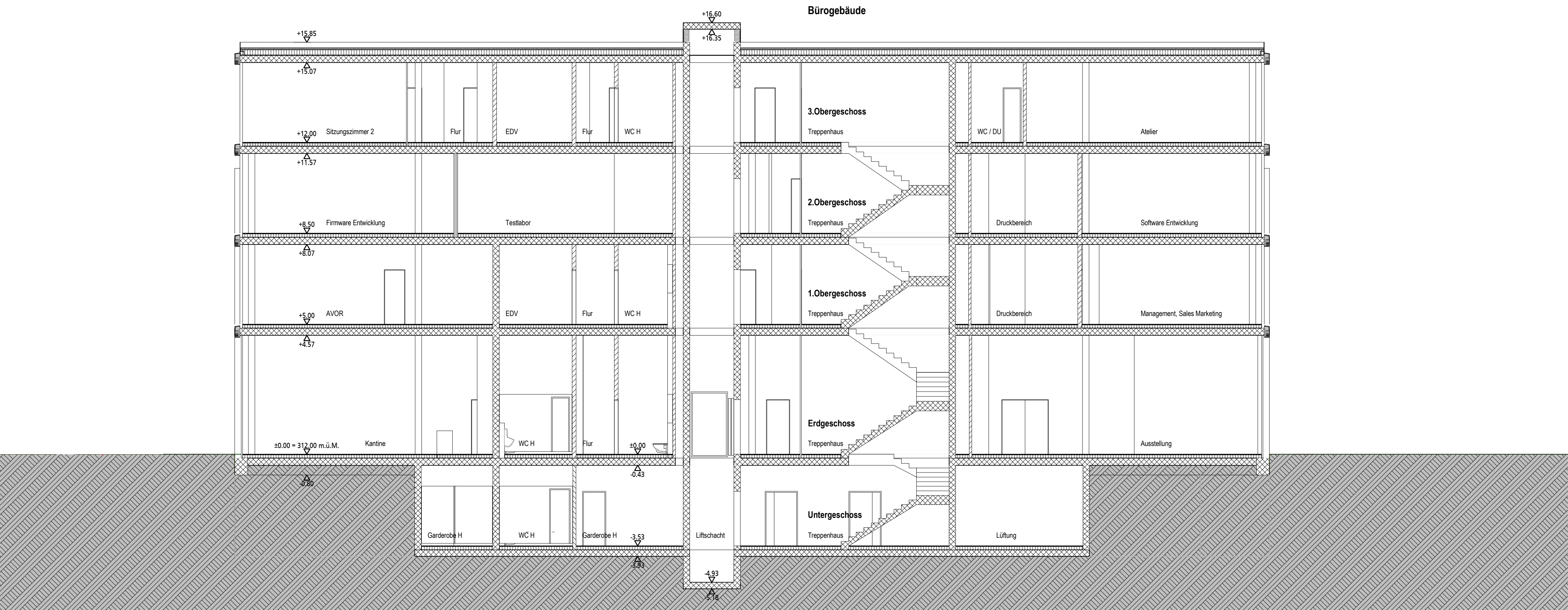
B - B | Querschnitt
